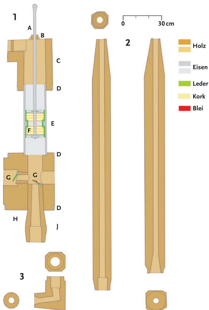
Abb. 9 Grube Gottesesegen. Schnitte durch Pumpe (1), Rohre (2) und Winkelstück (3) aus dem Bensbergs Gesenk. A: Kolbenstange; B: Kolbenstangenführung; C: Zylinderkopf; D: Metallreifen; E: Zylinder; F: Kolben; G: Druckventile; H: Pumpenunterteil; J: Saugstutzen (Grafik: LWL-Archäologie für Westfalen/M. Zeiler nach Planunterlagen des Wasserverbandes Siegen-Wittgenstein).
