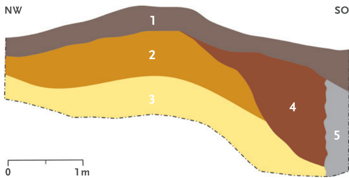
Abb. 4 Pingenfeld oberhalb der Grube Gottessegen. Profil des Pingenschnitts (Vermessung: LWL-Archäologie für Westfalen/E. Cichy, A. Knäpper, M. Zeiler; Grafik: LWL-Archäologie für Westfalen/M. Zeiler).
