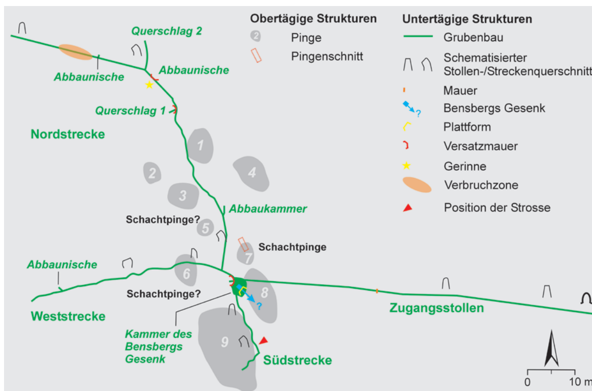
Abb. 3 Grube Gottessegen. Grundriss der oberen Sohle (Vermessung: LWL-Archäologie für Westfalen/E. Cichy, M. Zeiler; Grafik: LWL-Archäologie für Westfalen/M. Zeiler).
