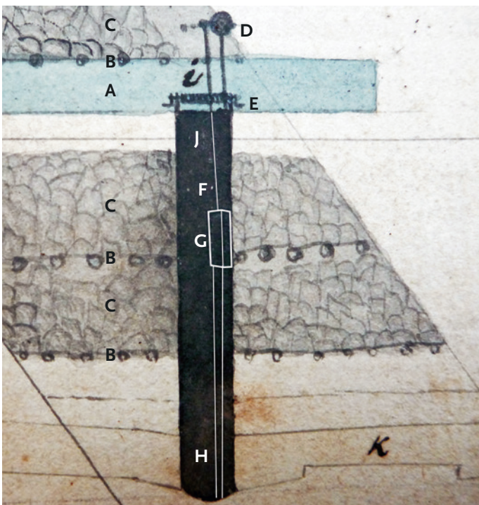
Abb. 11 Wasserförderung in einem Saigerriss der Grube Silberart von 1800. Die technischen Elemente sind zum besseren Verständnis weiß überzeichnet worden, da die Grafik im Original mit schwarzer Tusche auf schwarzem Hintergrund ausgeführt wurde. A: Strecke/Stollen; B: Bühne; C: Versatz; D: Bedienungseinrichtung für die Pumpe; E: Haspel; F: Gestänge; G: Pumpe; H: Rohre; J: Schacht (Archiv des Stahlbergmuseums Müsen).
