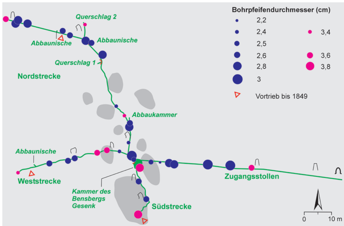
Abb. 17 Grube Gottessegen. Kartierung der Bohrpfefendurchmesser (Grafik: LWL-Archäologie für Westfalen/M. Zeiler).
