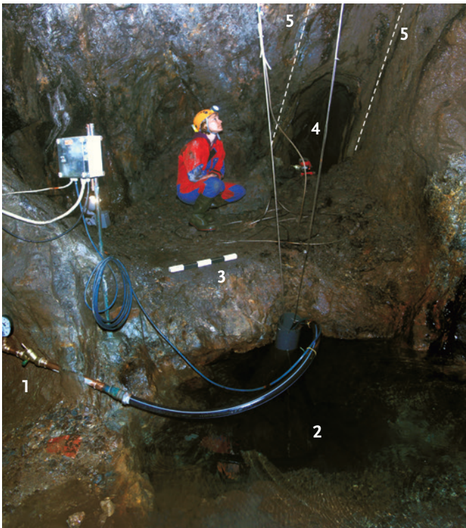
Abb. 7 Grube Gottessegen, Kammer des Bensbergs Gesenks. 1: Stolleneinmündung; 2: Blindschacht; 3: Plattform; 4: Südstrecke; 5: Schematisierte Grenzen der Gangzone (Foto: LWL-Archäologie für Westfalen/M. Zeiler).
