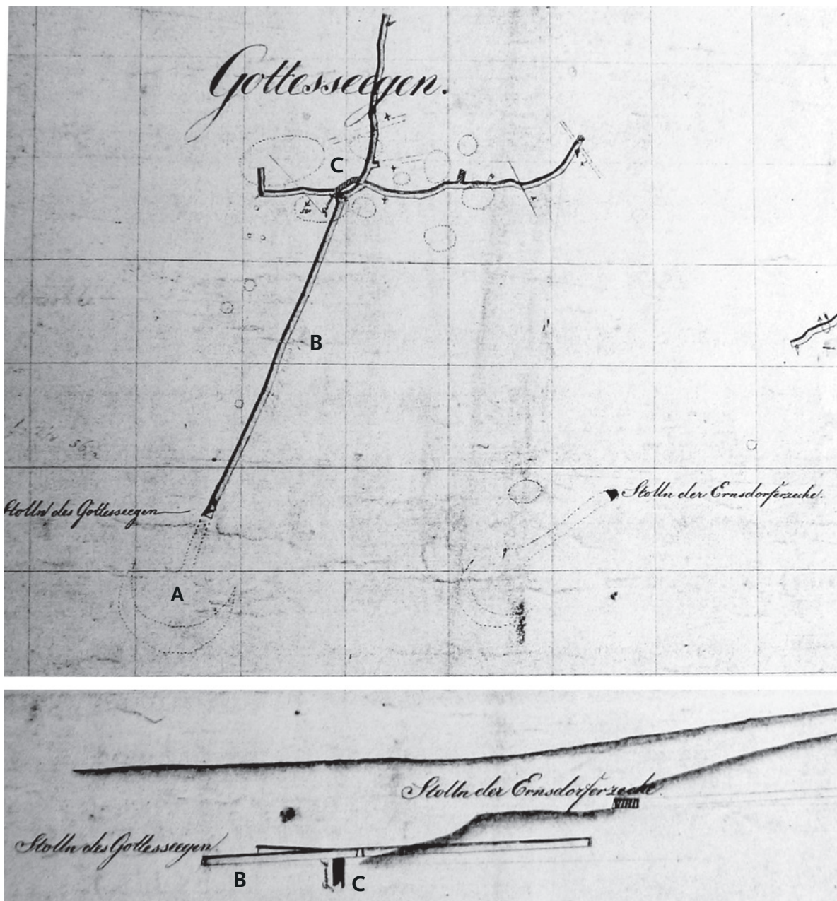
Abb. 20 Grube Gottessegen. 1834–1849 aktualisierter Grund- und Saigerriss. A: Heutiger Standort der Waldesruh Hütten; B: Zugangsstollen Gottessegen; C: Bensbergs Gesenk (Archiv des Stahlbergmuseums Müsen).
