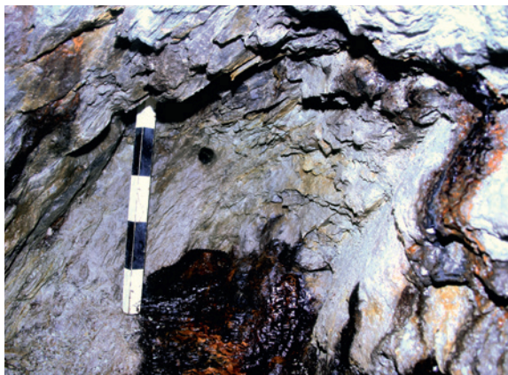
Abb. 18 Grube Gottessegen. Ortsbrust der Südstrecke mit Bohrpfefie (Foto: LWL-Archäologie für Westfalen/M. Zeiler).
