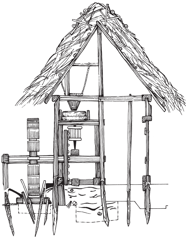
95 Ertstadt-Niederberg, Rotbachtal. Rekonstruktion einer merowingerzeitlichen Wassermühle aus Dasing bei Augsburg.
