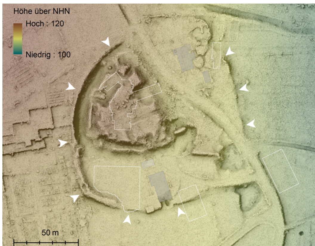
Abb. 2 Im Digitalen Geländemodell zeichnen sich die Reste der Burg Horstmar deutlich ab. Die weißen Pfeile markieren die mutmaßliche Ausdehnung der Vorburg. Weiß umrandet sind die mit Bodenradar prospektierten Flächen (Kartengrundlage: Land NRW [2022] – Lizenz dl-de/zero-2-0; Grafik: LWL-Archäologie für Westfalen/J. Coolen).
