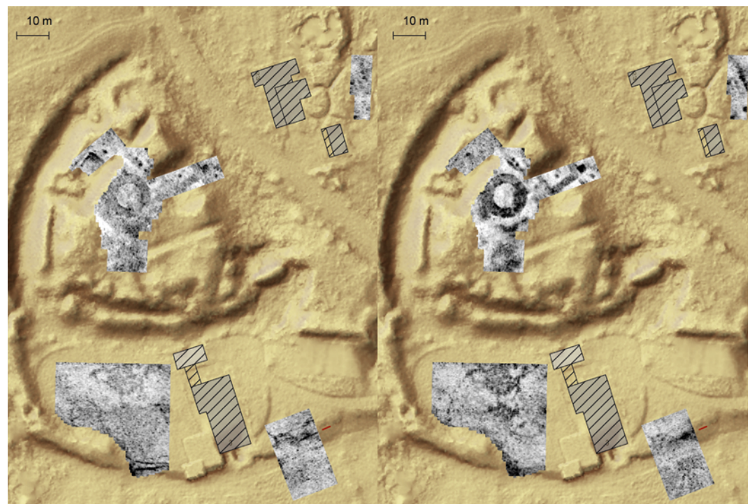
Abb. 3 Tiefscheiben der Bodenradarmessungen mit den Reflektionen in ca. 50–100 cm (links) bzw. 100–150 cm (rechts) Tiefe. Reflektierende Bereiche sind schwarz, absorbierende weiß dargestellt. Im Hintergrund (braun) eine aus dem Geländemodell abgeleitete Visualisierung der Geländestrukturen. Die kurze rote Linie rechts unten im Bild markiert den sichtbaren Teil einer mutmaßlichen Blendmauer (Kartengrundlage: Land NRW [2022] – Lizenz dl-de/zero-2-0; Grafik: LWL-Archäologie für Westfalen/J. Coolen).
