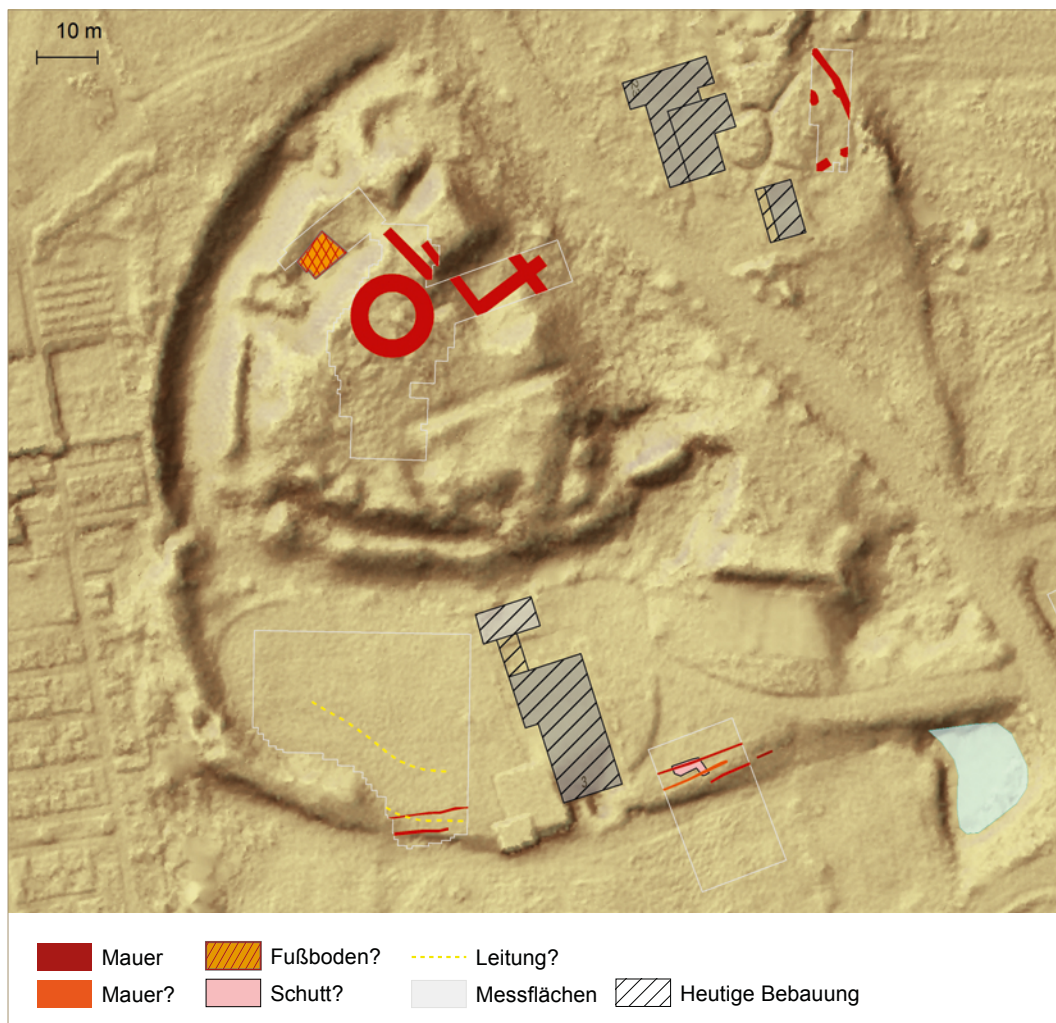
Abb. 4 Archäologische Interpretation der in den Radartiefenscheiben erkennbaren Strukturen (Kartengrundlage: Land NRW [2022] – Lizenz dl-de/zero-2-0; Grafik: LWL-Archäologie für Westfalen/J. Coolen).
