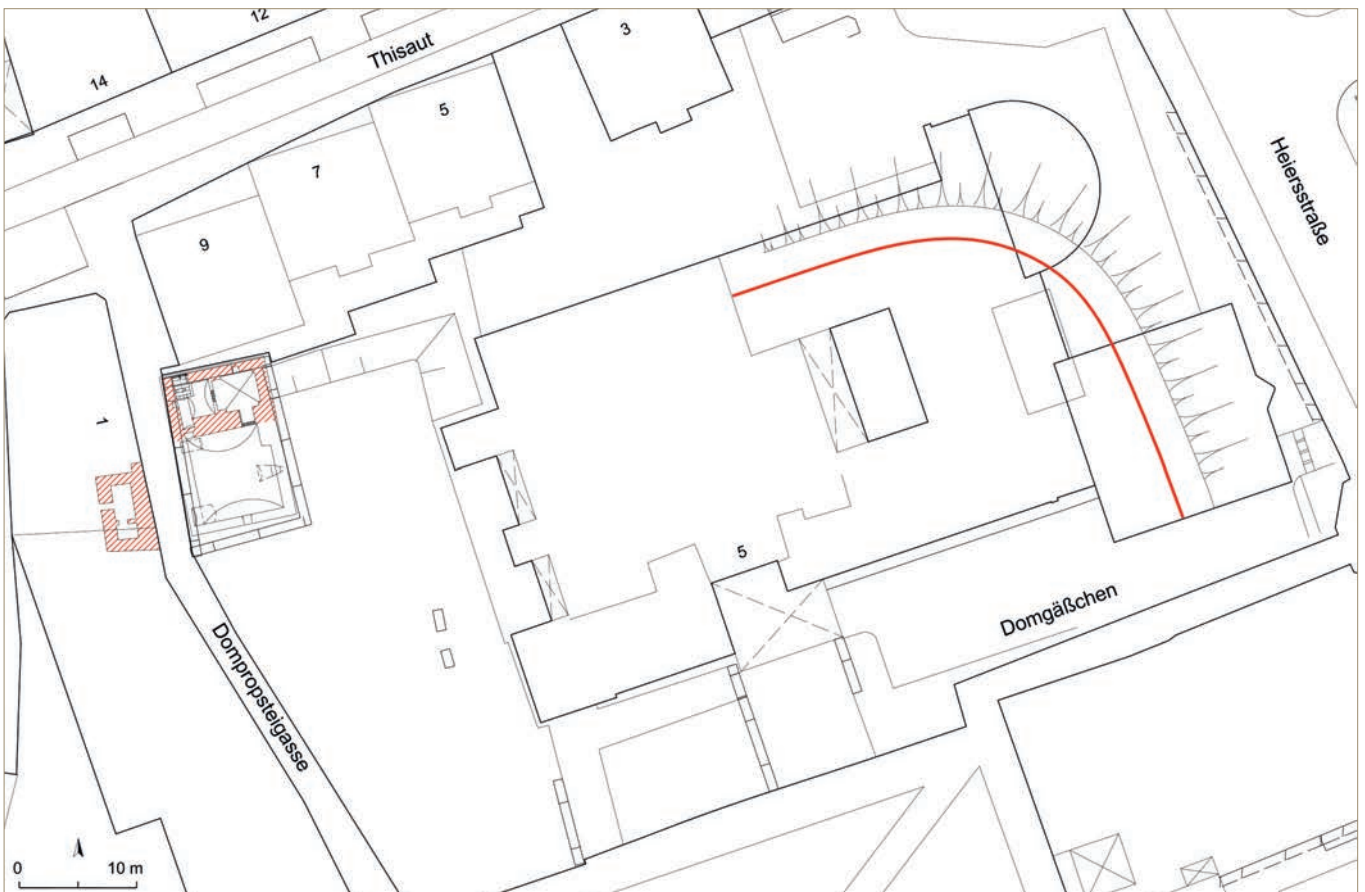
Abb. 5 Übersichtsplan vom Nordteil der Domburg mit den Flankierungsbauten beiderseits der ursprüng- lich mit einem Torbogen ver- sehenen Dompropsteigasse (Grafik: LWL-Archäolo- gie für Westfalen/O. Heil- mann, S. Spiong).
