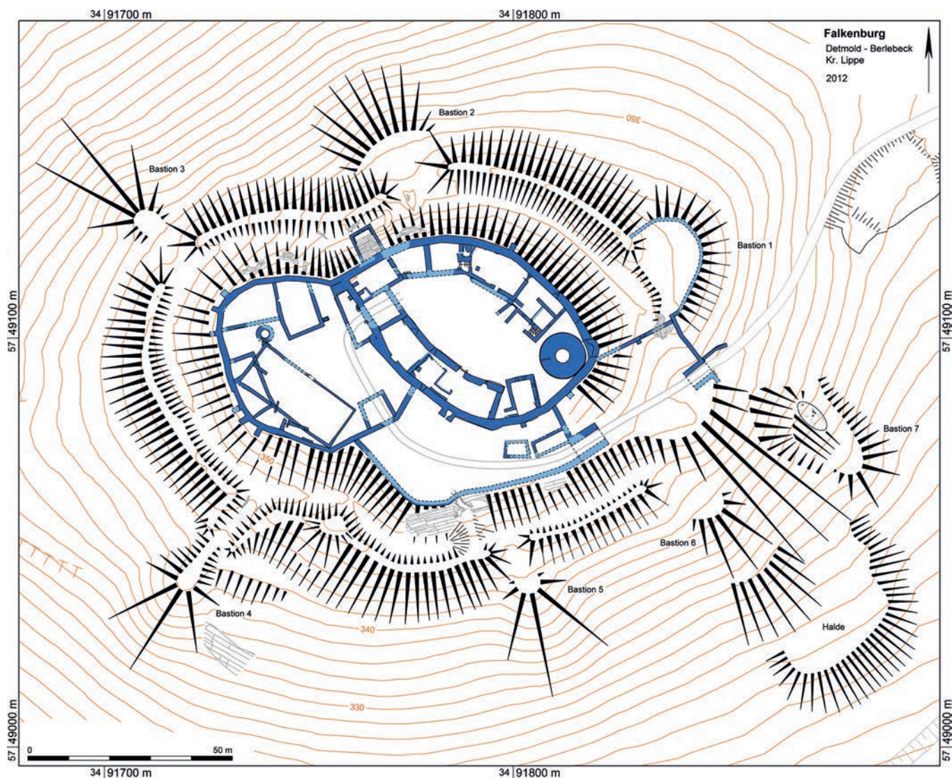
Abb. 2 Gesamtplan der mindestens dreiphasigen Gebäude- und Geländestrukturen der Falkenburg, Stand 2012 (Grafik: Vermessungs- und Zeichenbüro Thede).
