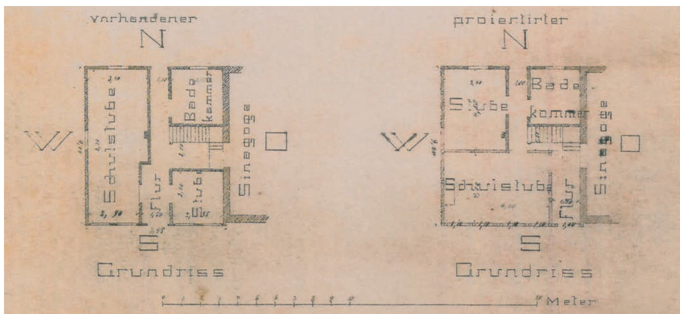
Abb.1 Skizze der jüdischen Schule mit dem Raumgefüge vor 1845/1846 (links) und nach dem geplanten Umbau von 1878 (rechts) (Plan: Stadtarchiv Petershagen, Amt Petershagen Nr. 199).
