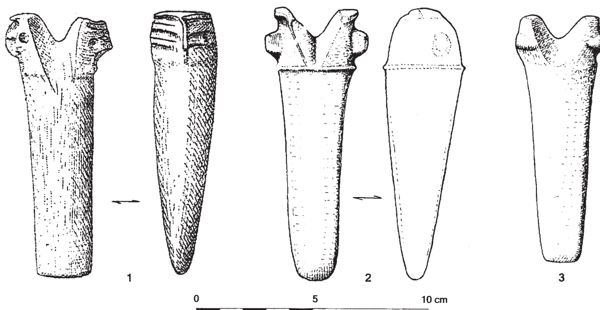
Fig. 5 Noyaux de moule pour haches à douille: 1 dépôt de Marlers (dép. Somme). – 2-3 dépôt de Thiais (dép. Val-de-Marne). – (Des-sins: 1 H. Breuil; 2-3 J.-P. Mohen).
