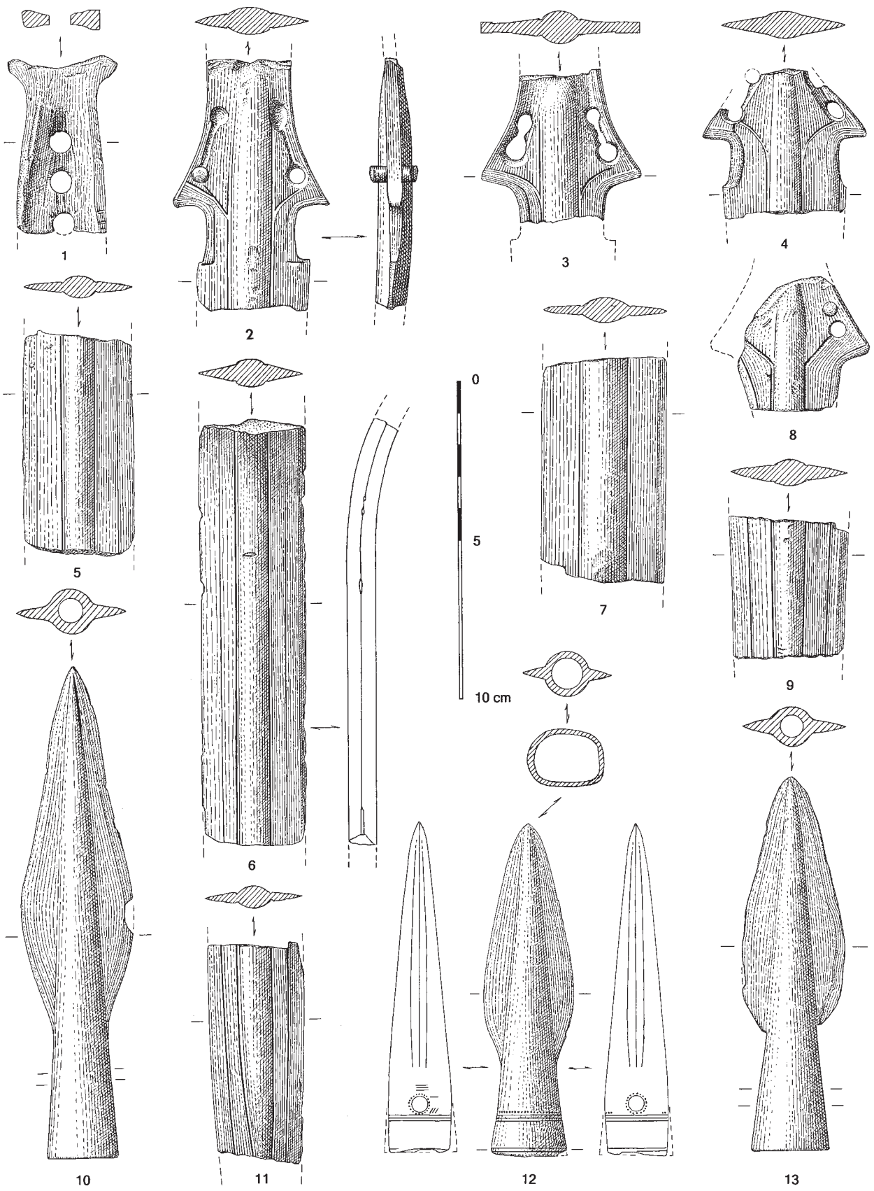
Fig. 3 Dépôt de Saint-Germain-sur-Vienne (dép. Indre-et-Loire): 1-9. 11 fragments d'épées. – 10. 12-13 pointes de lance. – (Dessins G. Cordier).
