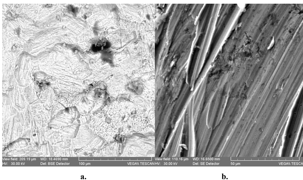
Fig. 3. Microfotografia SEM a brățării de fier de la Braniște: Structura de suprafață a patinei reziduale; b. Zona curățată mecanic.
