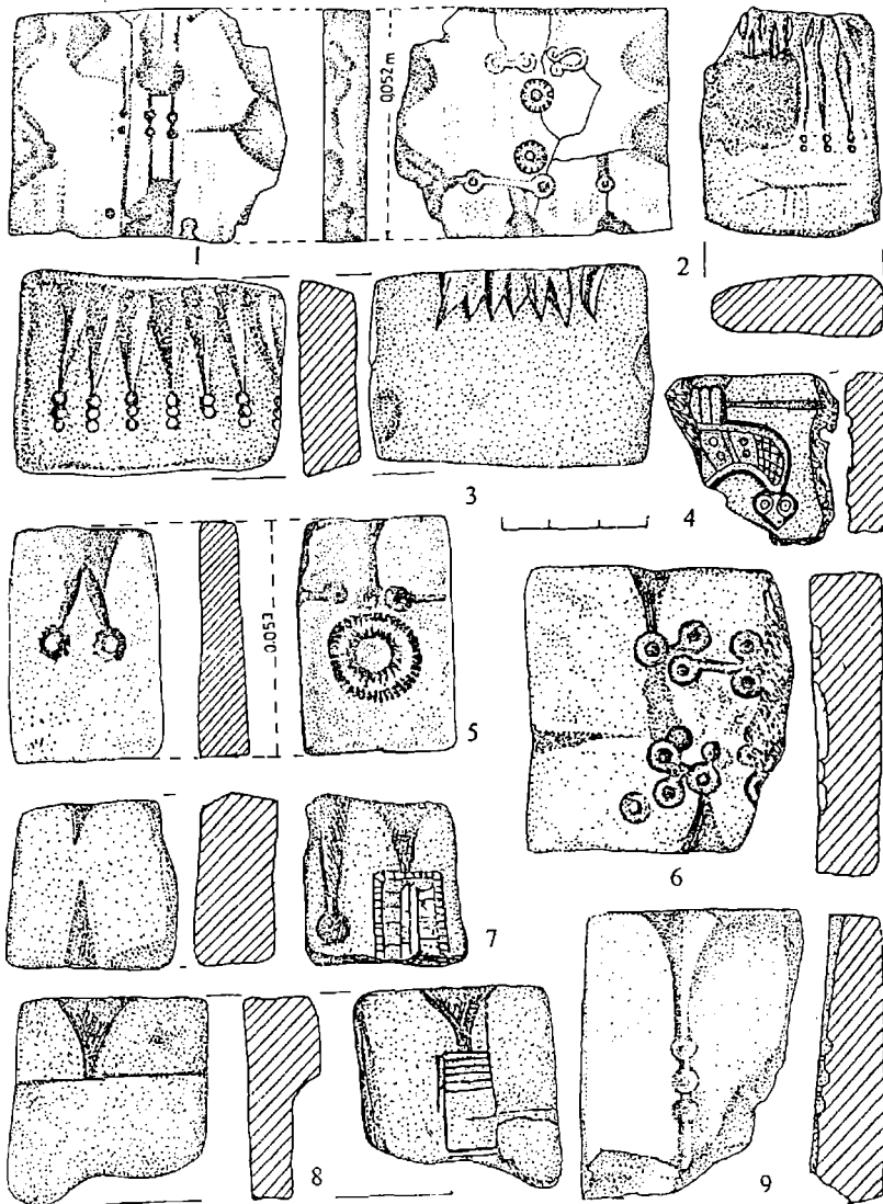
Fig. 2. Tipare din piatră pentru obiecte de podoabă 1. Ștefan cel Mare- Bacău; 2. Gura Idricii- Vaslui; 3. Seliște-Orhei; 4. Dobrinăuți-Cernăuți; 5. Moța-Iași; 6. Coroteni-Vrancea; 7-8. Dănceni-Ialoveni; 9. Dudești-Vaslui.
