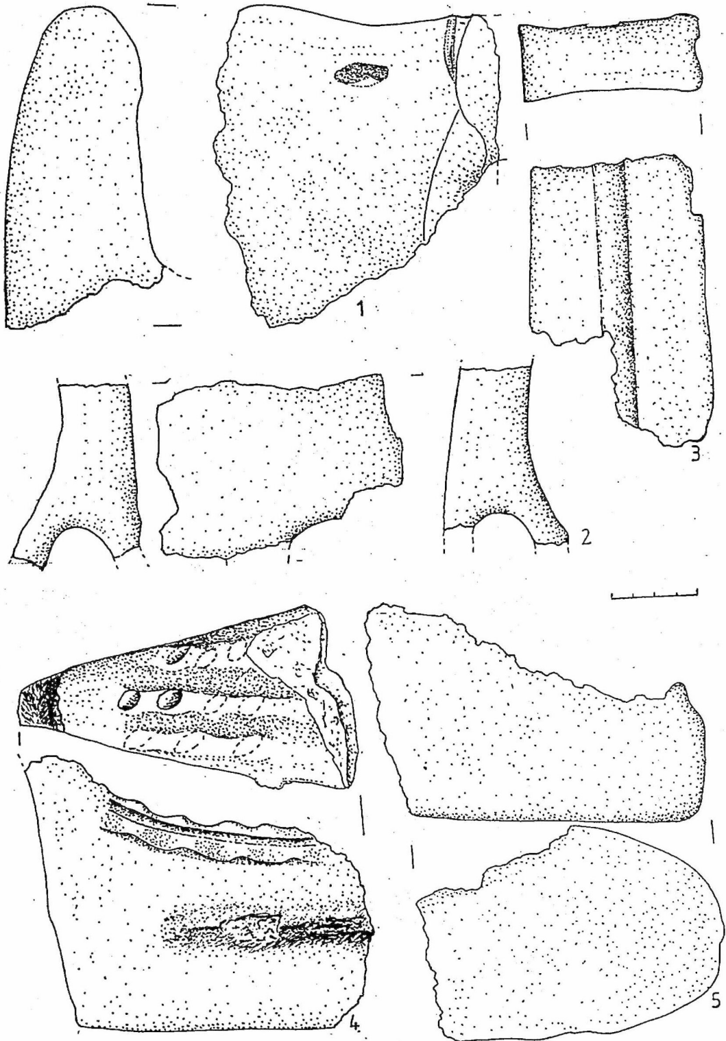
Fig. 53. Poiana. Căței de vatră din pământ ars.
