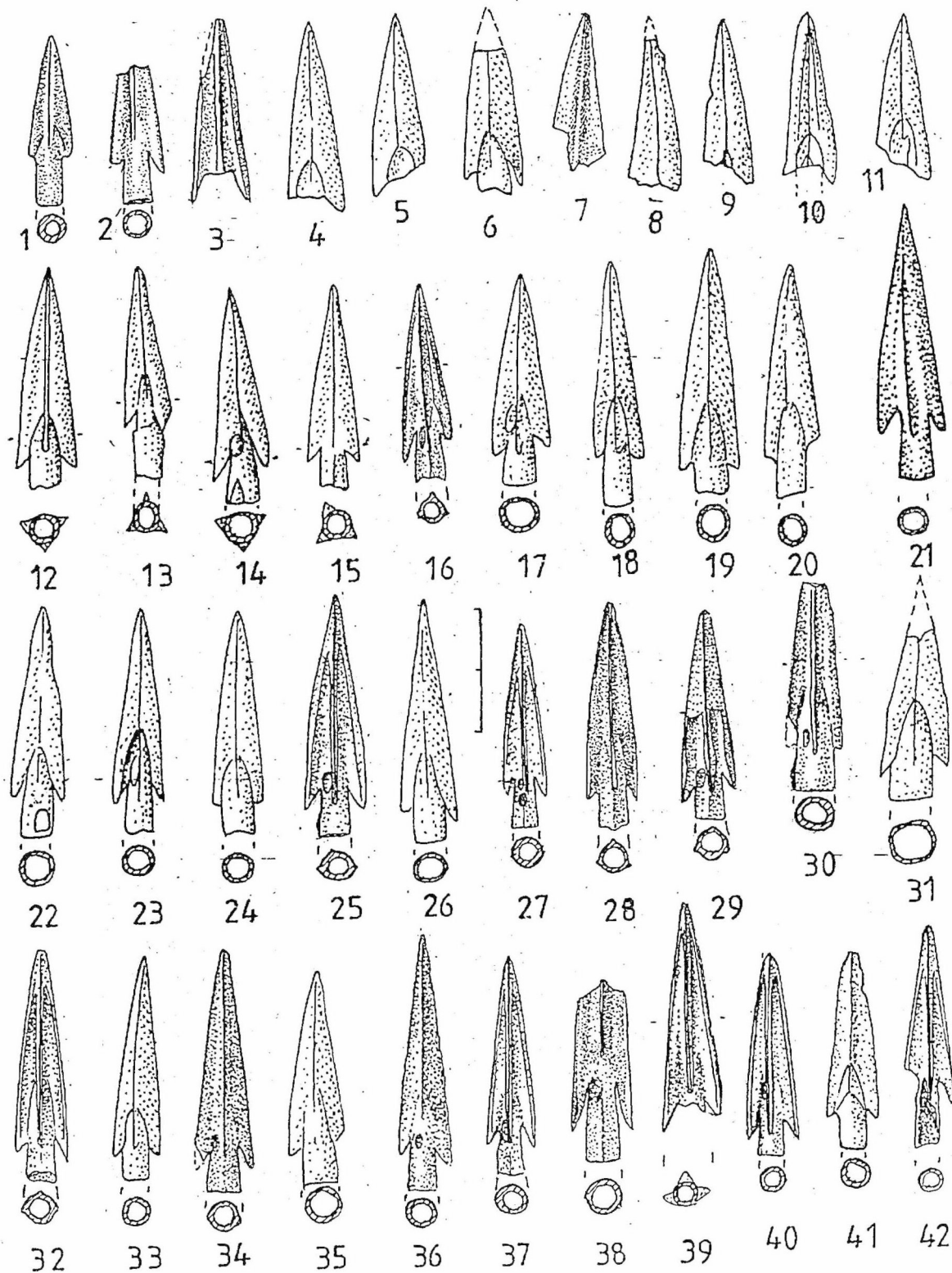
Fig. 41. Poiana. Vârfuri de săgeată de bronz.
