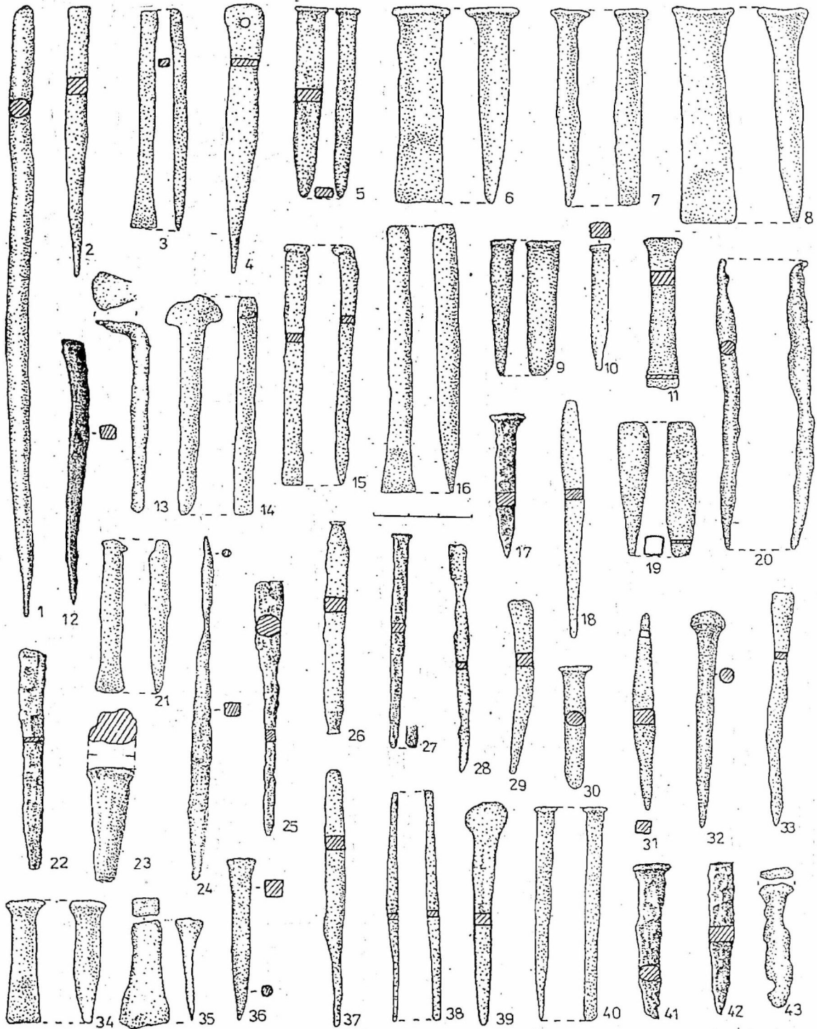
Fig. 14. Poiana. Dălți (3-4, 6-9, 11, 15-16, 19, 21, 27, 34-35, 40), străpungători (1-2, 12, 18, 20, 22, 24, 28-29, 31, 33, 37-38), dormuri (5, 10, 17, 23, 25-26, 30, 32, 36, 39, 41-43) și cuie (13-14) de fier.
