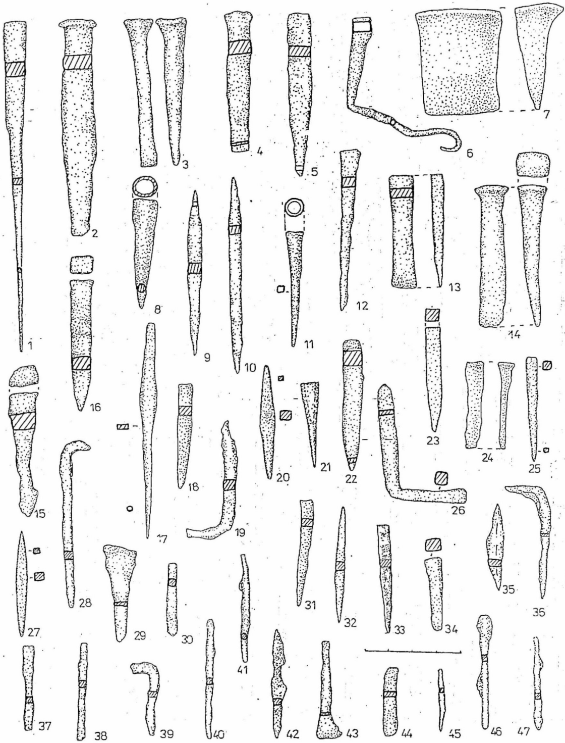
Fig. 15. Poiana. Dornuri (2, 5, 15-16, 22, 25, 34), străpungători (1, 6, 8-12, 17-18, 20-21, 23, 27-29, 31-33, 35, 40-42, 45), dălți (3-4, 13-14, 24, 43), nicovală (7), scoabe (19, 26, 36-37, 39), cui (30) și bare (38, 44, 46-47) de fier.
