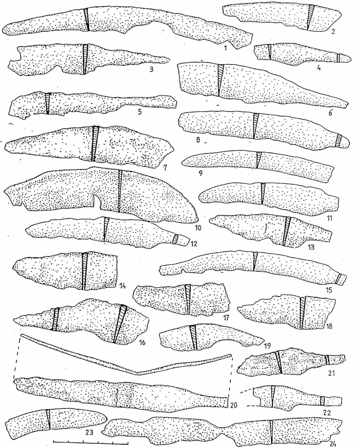
Fig. 6. Poiana. Seceri (1-2, 9, 15, 23), cosoare (4-8, 10-13, 16, 19, 21-22), pilă (20) și cuțite (3, 14, 17-18, 24) de fier.
