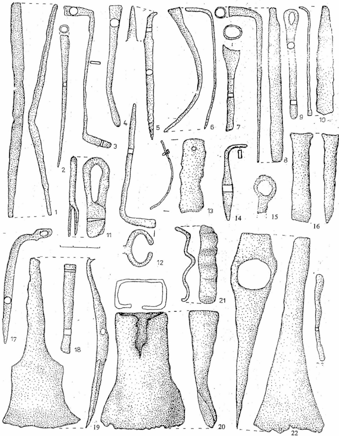
Fig. 3. Poiana. Pile (1, 8, 10), scoabe (3, 6, 12, 14), sule (2, 7), cheie (9), șurubelniță (5), foarfece (11), mâner (15), daltă (16), otic (19), topoare (20, 22), belciug (17), bare (4, 18, 23) și alte fragmente (13, 21) de fier.
