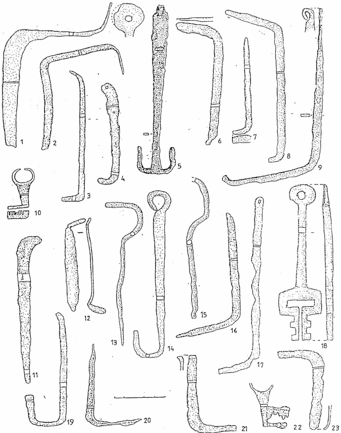
Fig. 2. Poiana. Chei (9-10, 18, 22), scoabe (2-3, 6-8, 11-12, 16, 19-21, 23), ivâr (5), încuietore (1), cârlige (13-15, 17) și garnitură (4) de fier.
