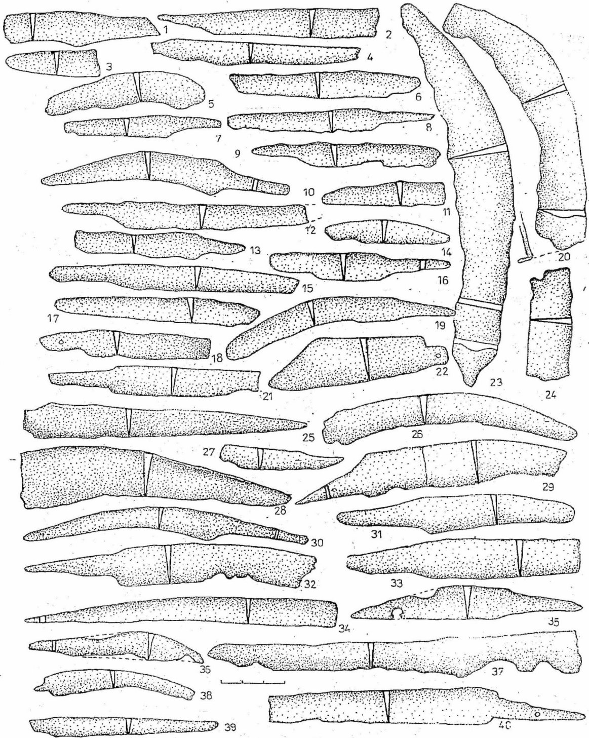
Fig. 7. Poiana. Cuțite (1-9, 11-13, 15-18, 21-22, 24-25, 27, 32-35, 37, 39-40), cosoare (10, 14, 19, 29-31, 36, 38) și seceri (20, 23, 26, 28) de fier.
