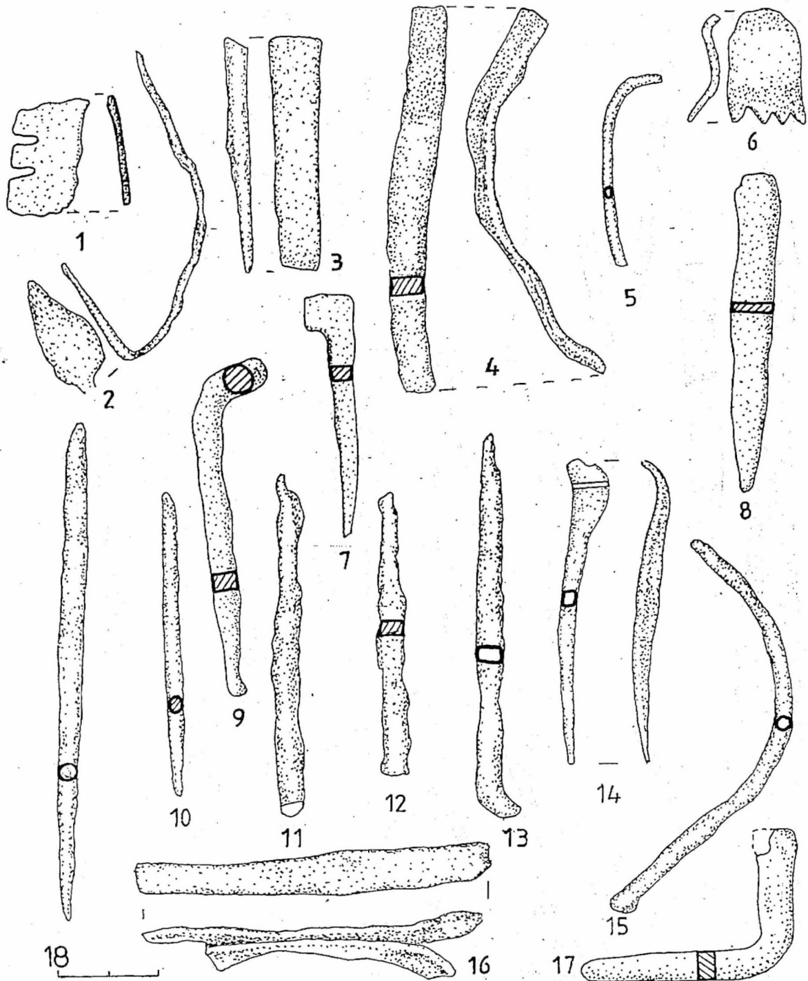
Fig. 19. Poiana. Fragmente de tablă (1, 6, 16), spatulă (2), daltă (3), sârmă (5, 15), pilă (8), scoabe (7, 13-14, 17), strâpungători (10, 12, 18) și bare (4, 9, 11) de fier.
