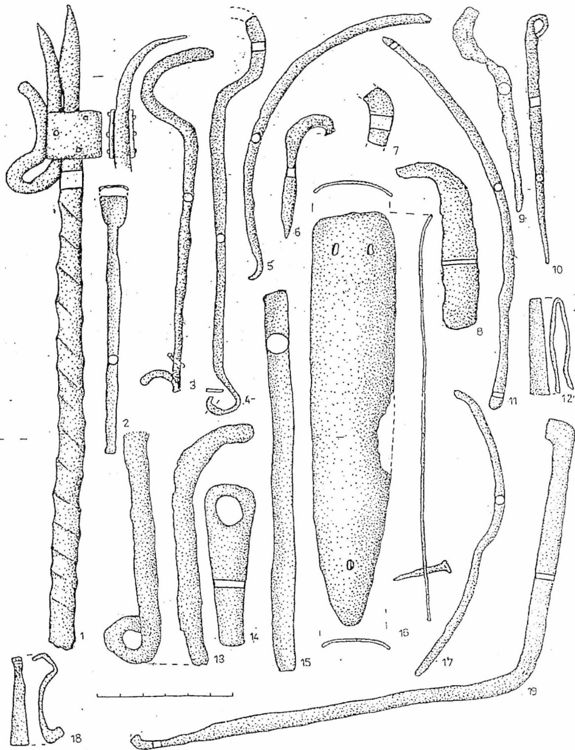
Fig. 12. Poiana. Furculiță (1), spatulă (2), cârlige (3-4, 18), mânere de cazan (5, 11), scoabă (6), clește (7, 9), pensetă (12), chcie (19), împungător (10) și diferite bare (8, 13-17) de fier.
