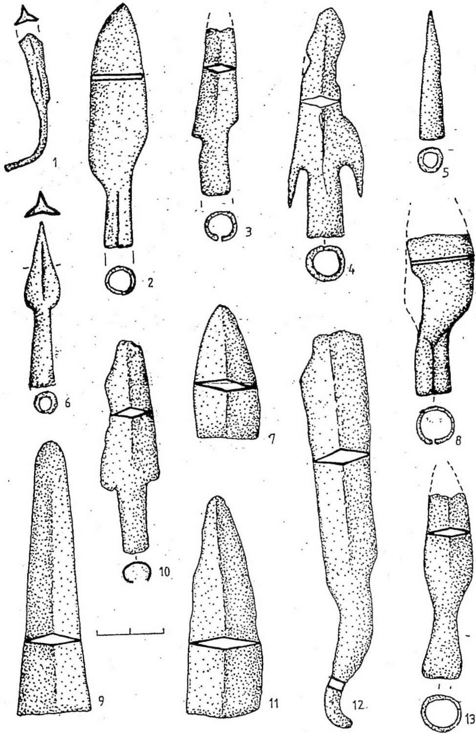
Fig. 37. Poiana. Vârfuri de lance și de săgeată, de fier.
