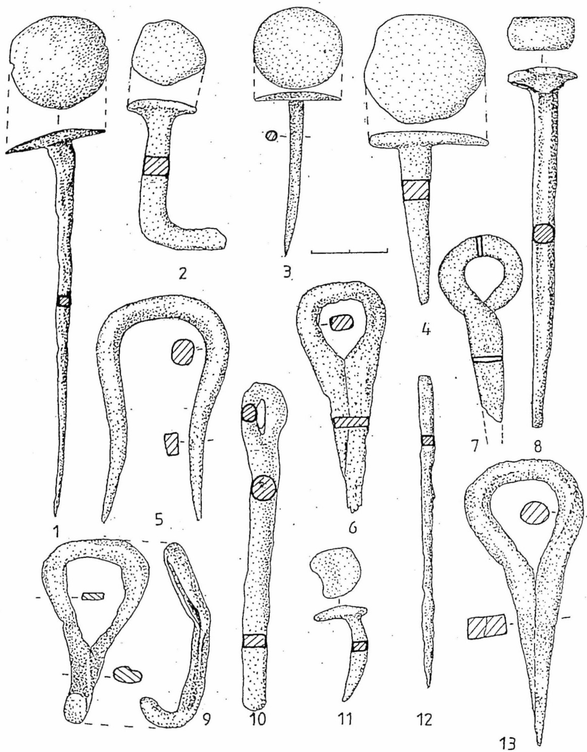
Fig. 24. Poiana. Piroane (1-2, 4, 8), cuie (3, 11), împungător (12), țâțâni (6, 9, 13), scoabă (5), încuietoare (7) și bară (10) de fier și bronz (3).
