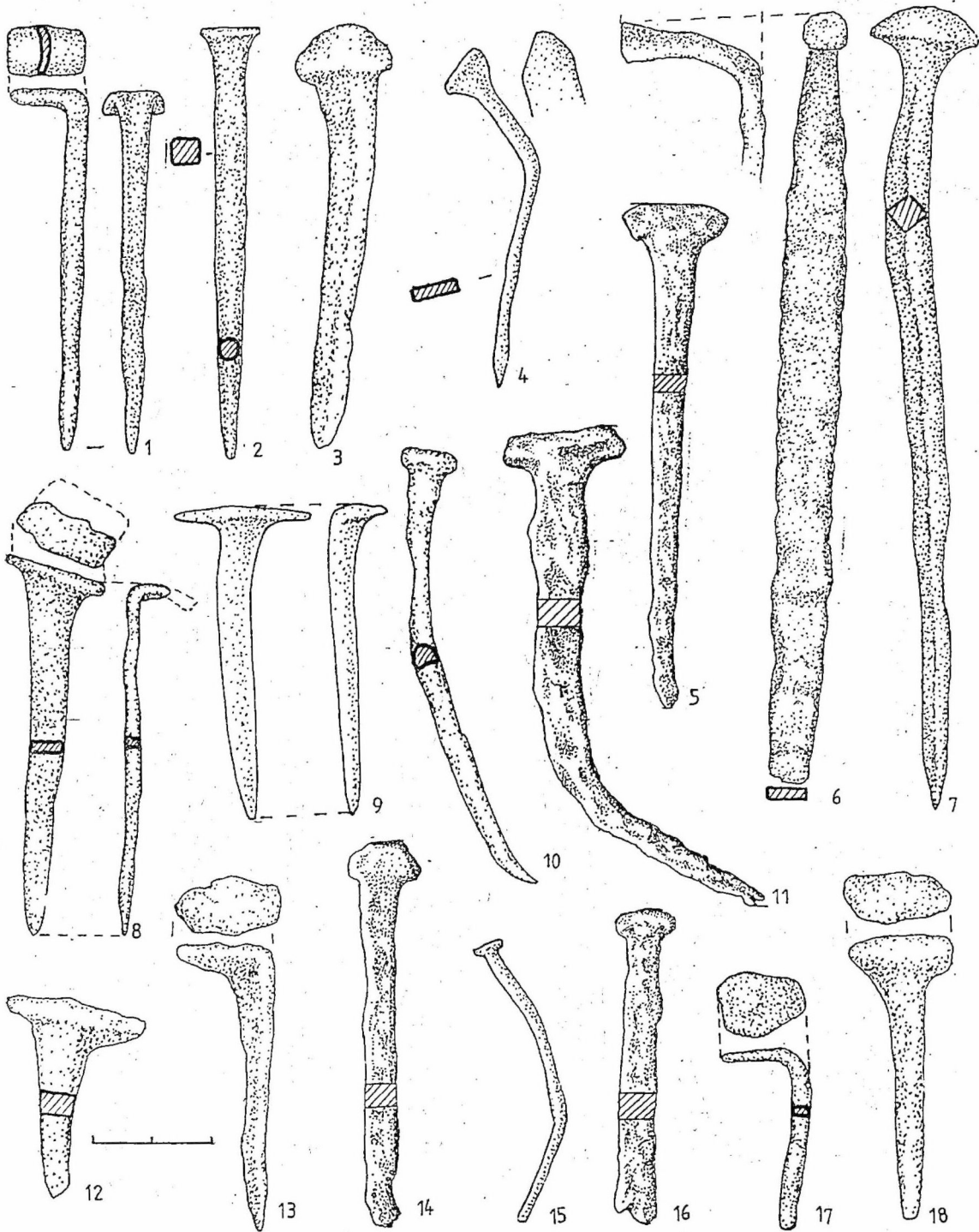
Fig. 25. Poiana. Cuie (1, 15), dornuri (2-3, 14, 16, 18), daltă (4, 17), piroane (5, 7-13) și pilă (6) de fier.
