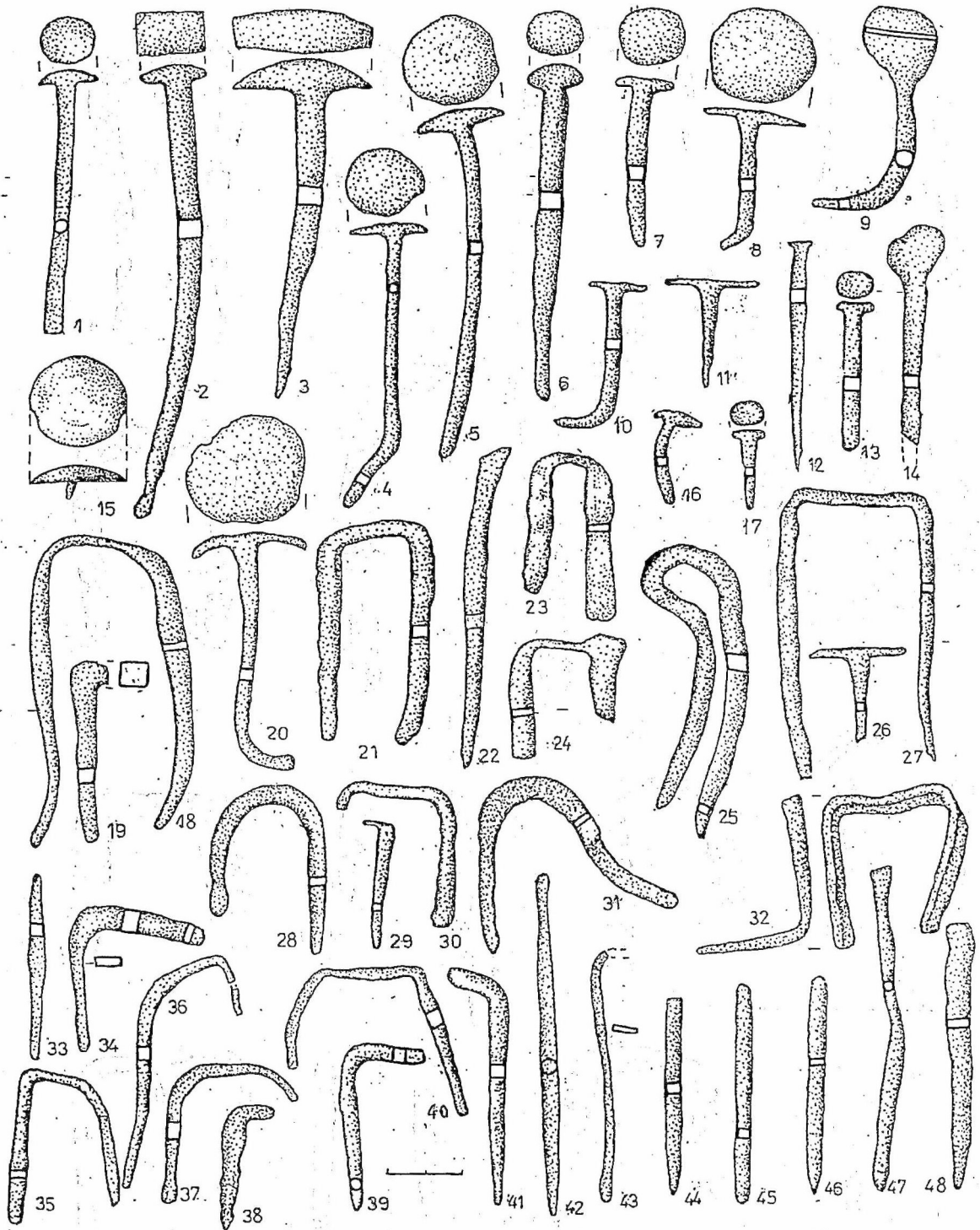
Fig. 28. Poiana. Cuie (1-2, 4-11, 15-16, 20, 26), piron (3), dormuri (12-14, 17), scoabe (18-19, 21-25, 27-32, 34-41, 48) și împungători (33, 42-47) de fier.
