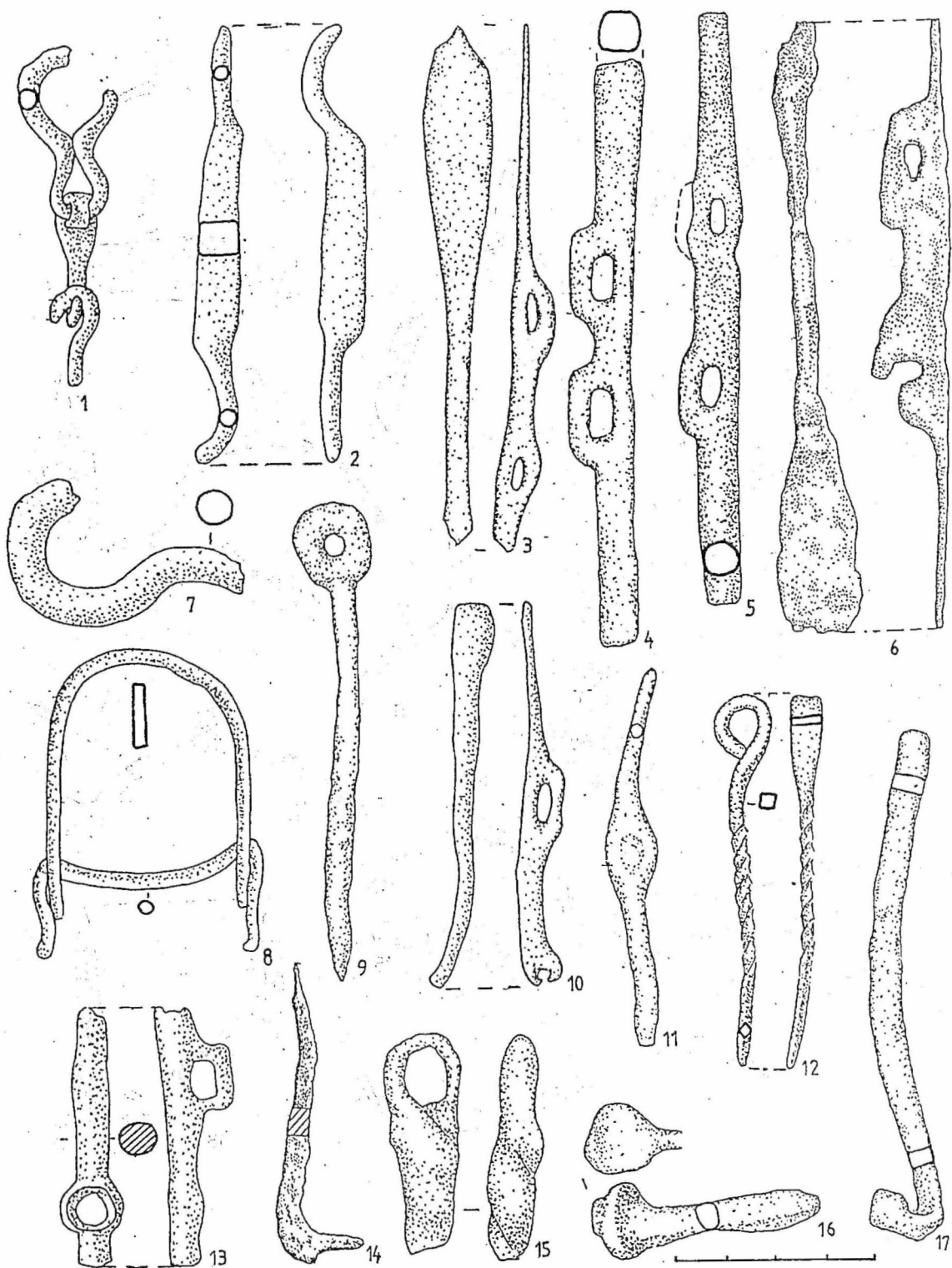
Fig. 30. Poiana. Piese de harnașament de fier.
