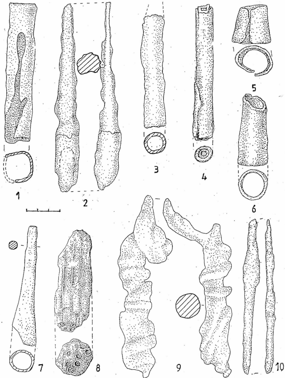
Fig. 36. Poiana. Fragmente de vârfuri și teci de lance de fier.
