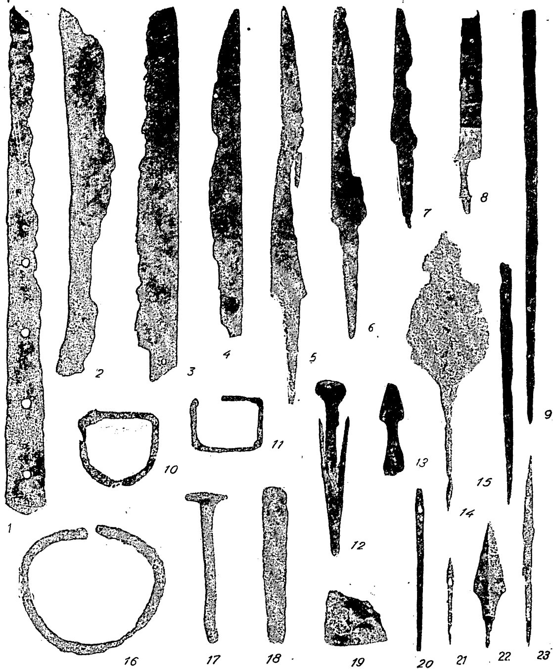
Fig. 3. — Obiecte de fier descoperite în bordeiele 1 (6—8, 21—23), 2 (3, 14) și 3 (1, 2, 4, 9—13, 15, 20), precum și în apropierea lor (5, 16—19).
