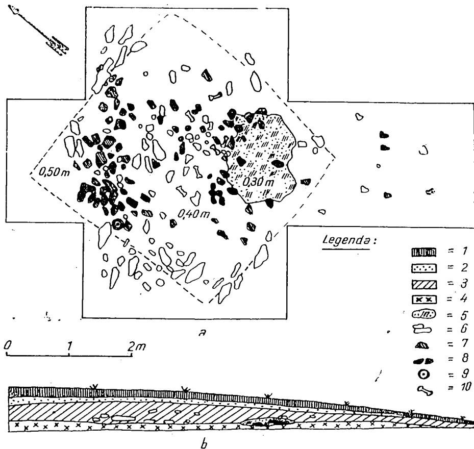
Fig. 1. — Planul (a) și profilul (b) locuinței de suprafață din așezarea Latène de la Șorogari. 1, sol arabil; 2, nivel prefeudal; 3, nivel Latène; 4, sol viu; 5, resturi de vatră; 6, resturi de chirpici; 7, fragmente ceramice; 8, pietre arse; 9, fusaiolă; 10, oase de animale.
