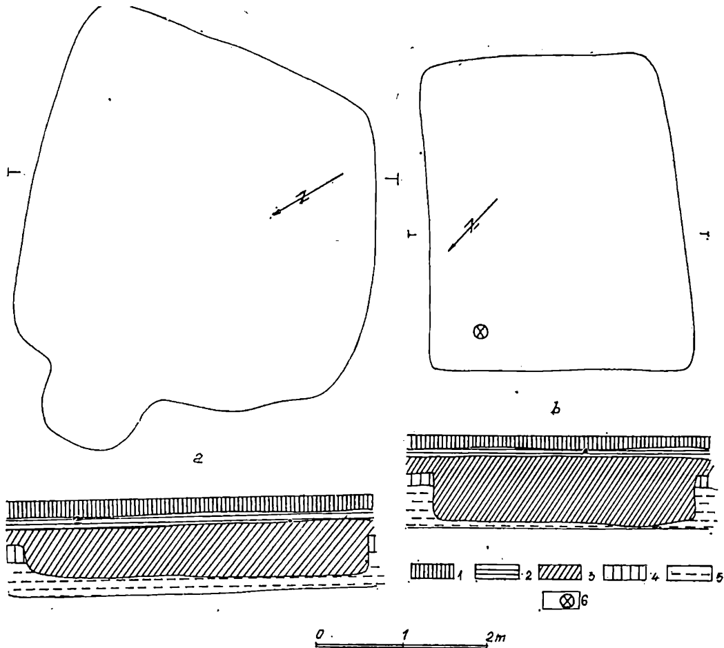
Fig. 12. — Planul și profilul bordeiilor 7 (a) și 8 (b): 1, sol vegetal; 2, strat din secolele VI — VII c.n.; 3, bordei din secolele II—III c.n.; 4, strat din a doua epocă a fierului; 5, sol virgin; 6, monedă.
