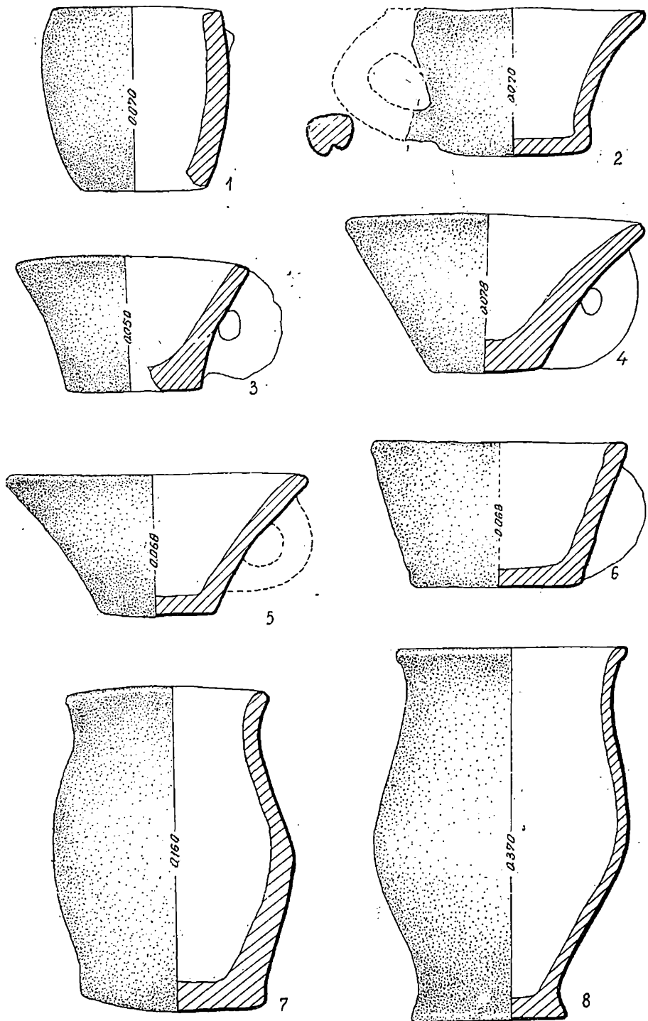
Fig. 45. — Ceramică lucrată cu mâna din așezarea din secolele II—III e.n.: 1, bordeiul 16; 2, 7, bordeiul 25; 3, bordeiul 22; 4, bordeiul 11; 5, bordeiul 24; 6, bordeiul 23; 8, bordeiul 12.
