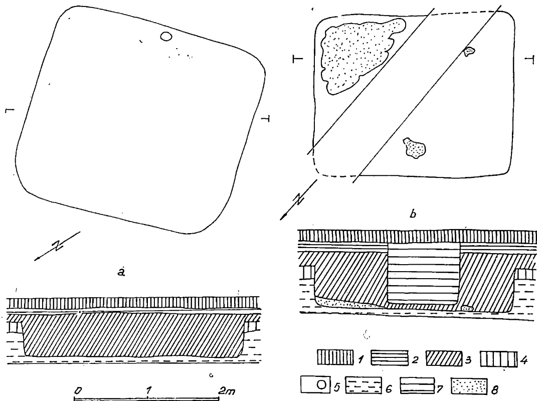
Fig. 11.—Planul și profilul bordeciilor 3 (a) și 5 (b): 1, sol vegetal; 2, strat din secolele VI—VII; 3, bordei din secolele II—III e.n.; 4, strat din a doua epocă a fierului; 5, groapă de par; 6, sol virgin; 7, șanț contemporan; 8, resturi de vatră.
