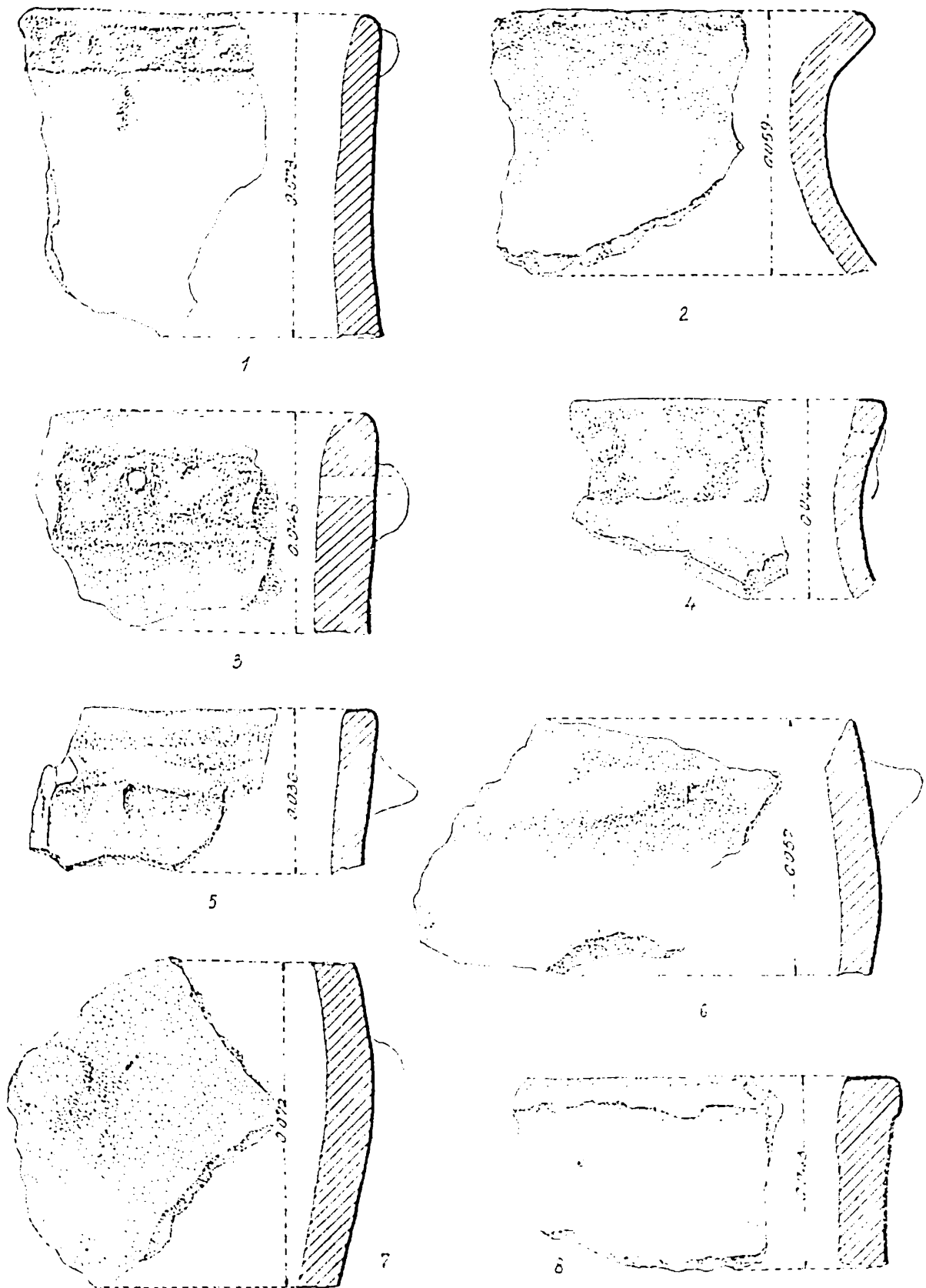
Fig. 26. — Ceramică lucrată cu mîna din așezarea Latène: 1-6, 8, bordeiul 13; 7, bordeiul 14.
