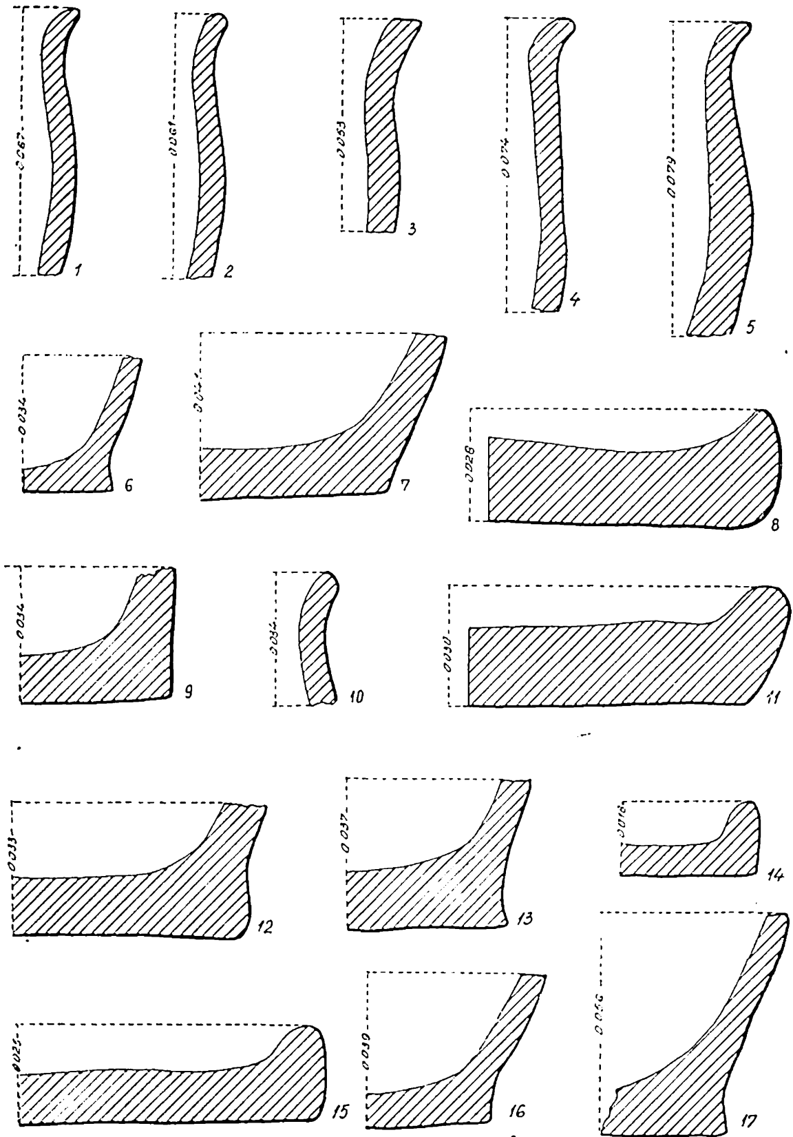
Fig. 60. — Ceramcă din așezarea din secolele VI–VII e.n.: 1, 2, 10, 15, 17, bordeiul 20; 3, 4, 7–9, 11, 14, bordeiul 19; 5, 6, 13, bordeiul 17; 12, 16, bordeiul 2.
