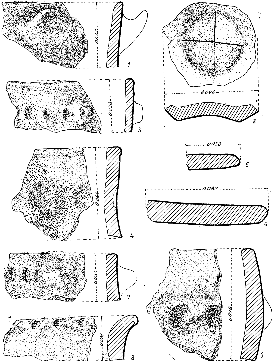
Fig. 23. — Ceramică lucrată cu mina din așezarea Latène: 1, 3, 5, 6, 9, bordeiul 10; 4, 7, 8, bordeiul 1; 2, bordeiul 6.
