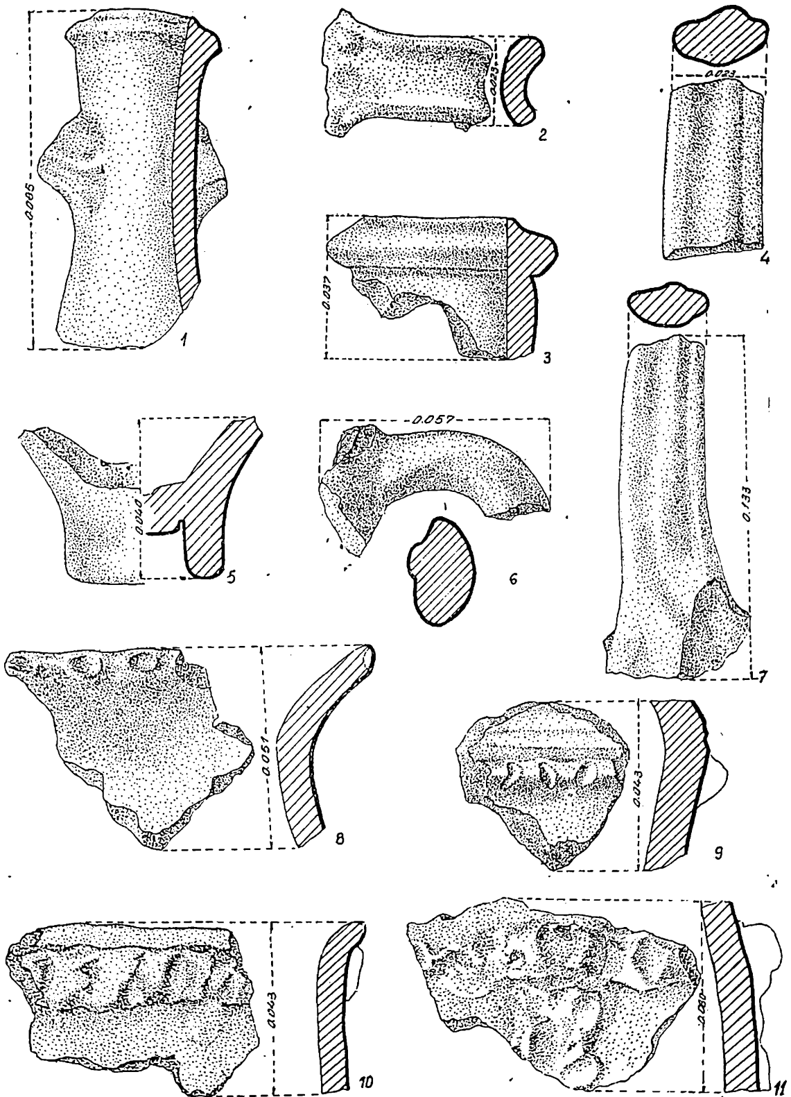
Fig. 41. — Ceramică lucrată cu mîna (8—11) și ceramică de import (1—7) din așezarea din secolele II—III e.n.: 1, 2, bordeiul 5; 3, 5, bordeiul 3; 4, bordeiul 8; 6, bordeiul 12; 7, bordeiul 11; 8, locuința 3; 9, bordeiul 9; 10, locuința 17; 11, locuința 9.
