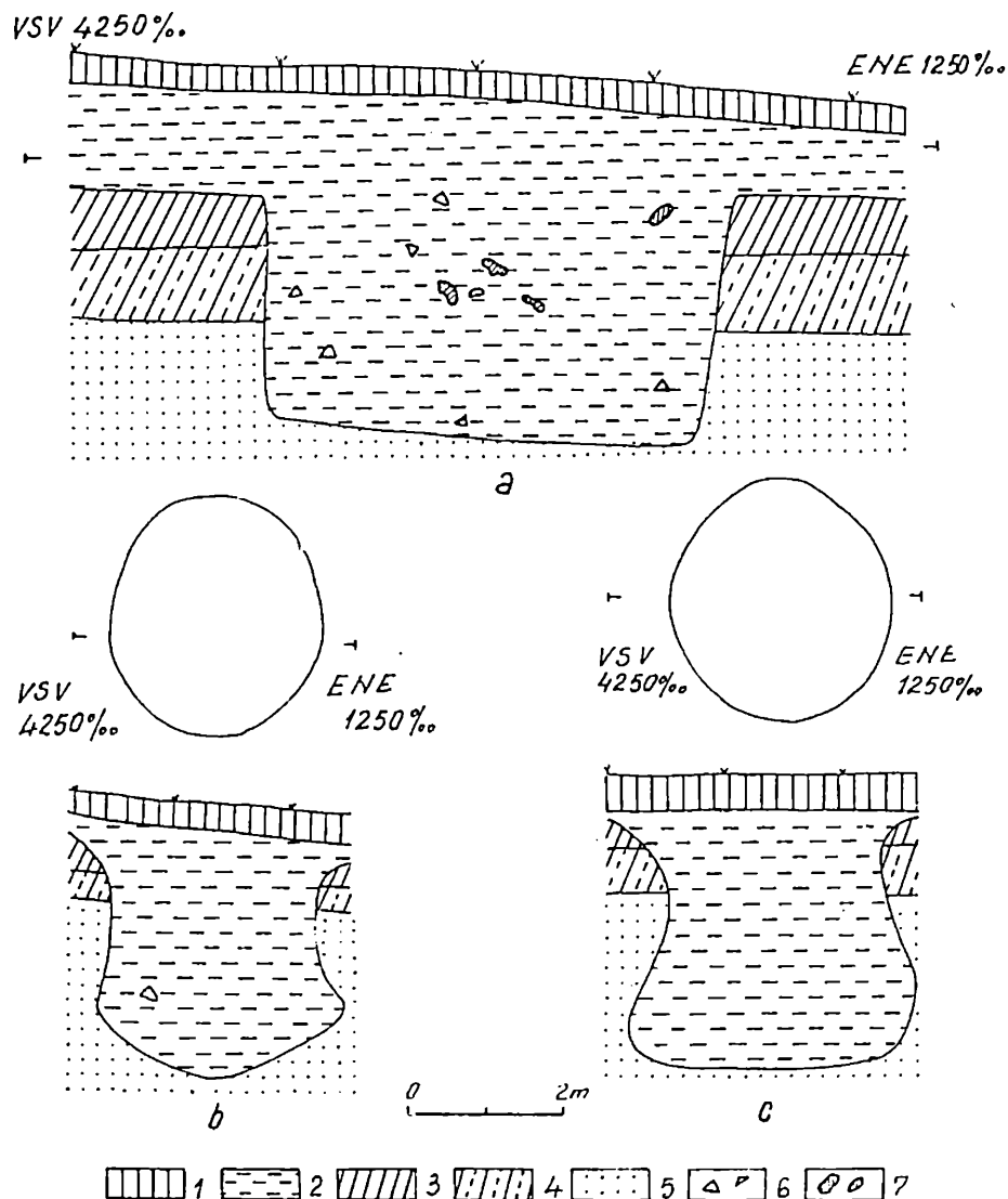
Fig. 1. — Locuință 28 (a) și gropile 52 (b) și 82 (c): 1, sol vegetal; 2, sol negru feudal (secolele XIV—XV); 3, sol brun-cenușos (secolul IV e. n.); 4, sol cafeniu (secolele II—III e.n.); 5, sol galben; 6, fragmente ceramice; 7, pietre.
