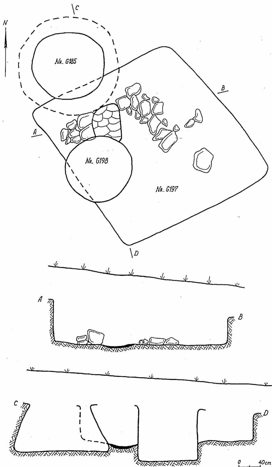
Fig. 4. Locuința nr. G197 din secolul IX și gropile menajere nr. G185, G198 din secolele X-XIII.
