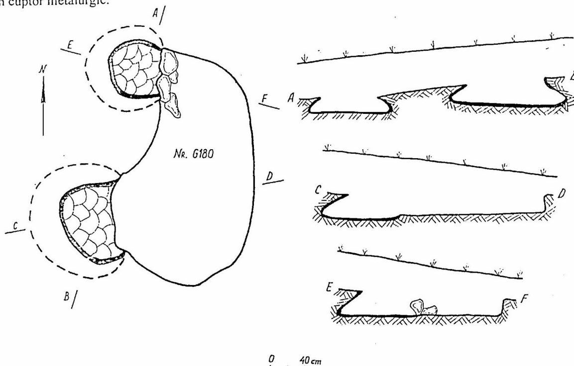
Fig. 8. Complexul meșteșugăresc nr. G180 din secolele VIII-IX.
