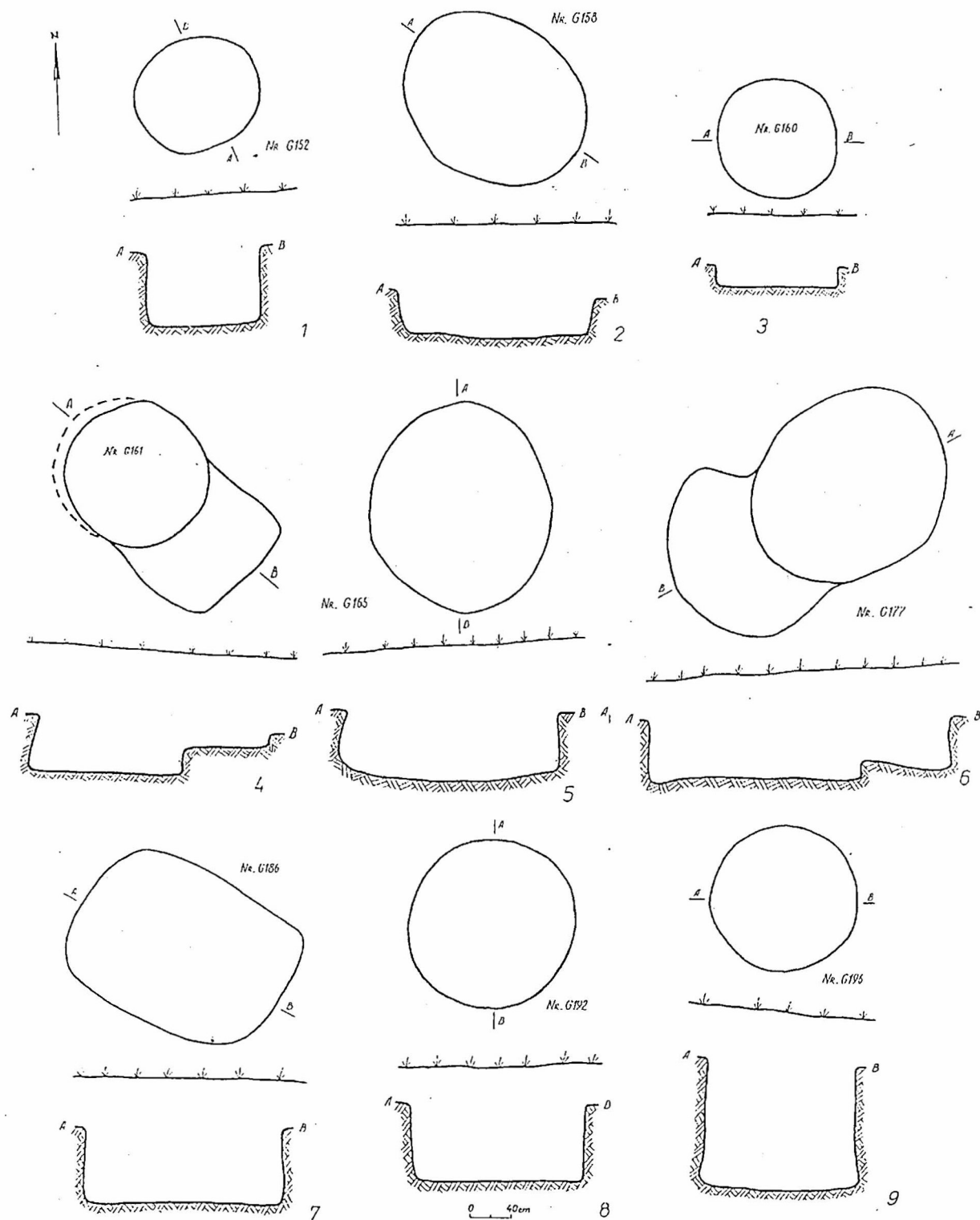
Fig. 2. Gropi menajere geto-dace din secolele IV-III î. de H. (1 – nr. G152, 2 – nr. G158, 3 – nr. G160, 4 – nr. G161, 5 – nr. G165, 6 – nr. G177, 7 – nr. G186, 8 – G192, 9 – nr. G196).
