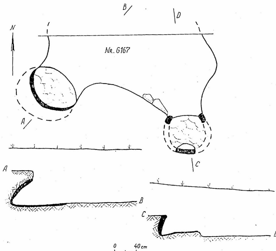
Fig. 6. Complexul meșteșugăresc nr. G167 din secolele VIII-IX.
