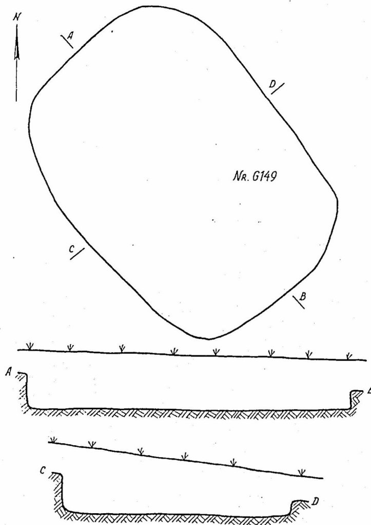
Fig. 10. Ancxa nr. G149 din secolele X-XIII.
