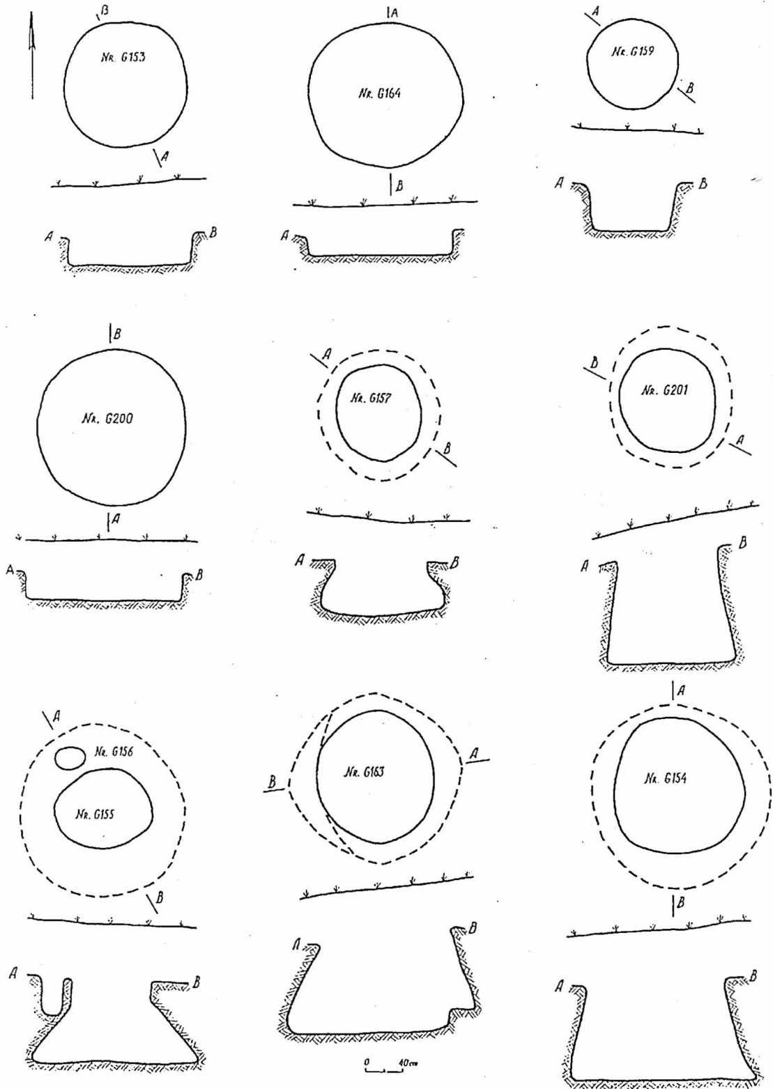
Fig. 12. Gropi menajere din secolele X-XIII: 1 - nr. G153; 2 - nr. G164; 3 - nr. G159; 4 - nr. G200; 5 - nr. G157; 6 - nr. G201; 7 - nr. G155; 8 - nr. G163; 9 - nr. G154.
