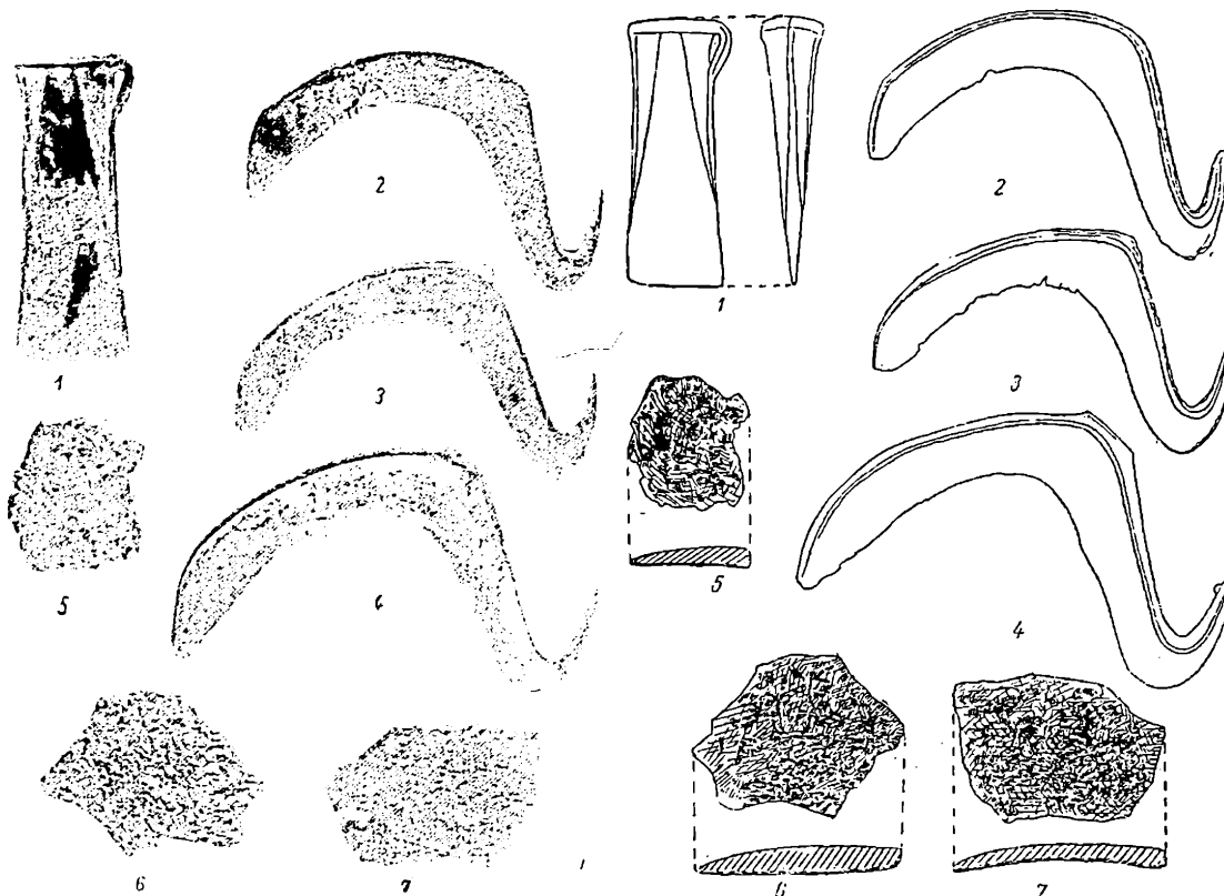
Fig. 1. — Depozitul de obiecte de bronz de la Bozia-Nouă. 1, celt; 2—4, seceri cu cârlig; 5—7, bucăți de turte de bronz (cca 1/3 m. nat.).
