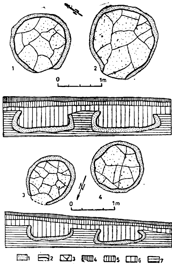
Fig. 6. Cuptoarele simple de ars ceramică, nr. 1—2 (1—2) și nr. 4—5 (3—4), plan și profil. 1, pămînt înroșit; 2, lipitură; 3, vatră; 4, sol vegetal; 5, nivel feudal, secolele XV—XVII; 6, nivel feudal timpuriu; 7, sol galben steril.
