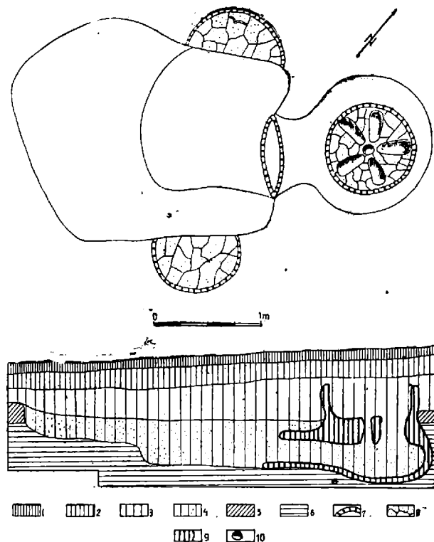
Fig. 5. Cuptorul de ars ceramică, nr. 7, plan și profil stratigrafic. 1, sol vegetal; 2, nivel feudal, secolele XV—XVII; 3, nivel feudal timpuriu; 4, umplutura gropii olarului; 5, nivel preistoric; 6, sol galben steril; 7, limita cuptoarelor; 8, lipitură de vatră; 9, pământ înroșit; 10, orificii de grătar.
