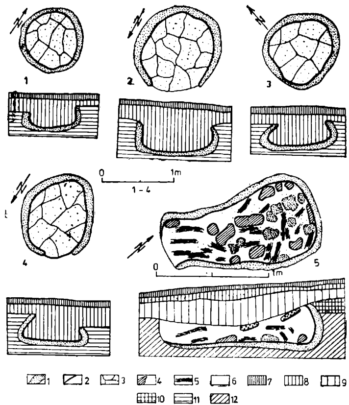
Fig. 7. Cuptoarele de copt piine nr. 3 (1), nr. 6 (2), nr. 11 (3) și nr. 9 (4) și cuptorul de prelucrat metale, nr. 12 (5), plan și profil. 1, pămînt înroșit; 2, lipitură; 3, vetre; 4, pietre; 5, lemn carbonizat; 6, zgură de fier; 7, sol vegetal; 8, nivel feudal secolele XV—XVII; 9, nivel feudal timpuriu; 10, nivel preistoric; 11, sol galben steril; 12, sol calcaros.
