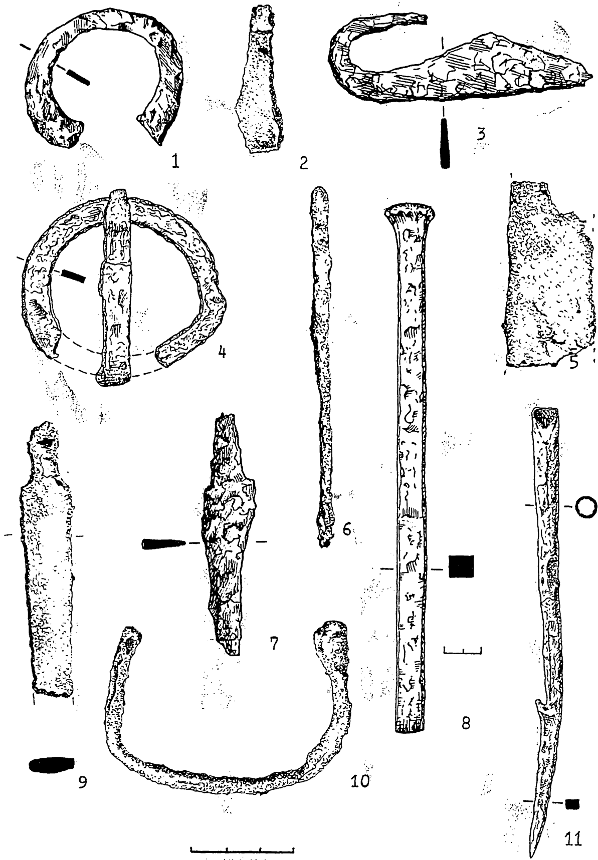
Fig. 5. Unele și obiecte vestimentare din fier: 2 – locuința 17; 5-6, 8-9 – locuința 22; 1, 3-5, 10 – locuința 23; 7 – locuința 25; 11 – strat cultural.
