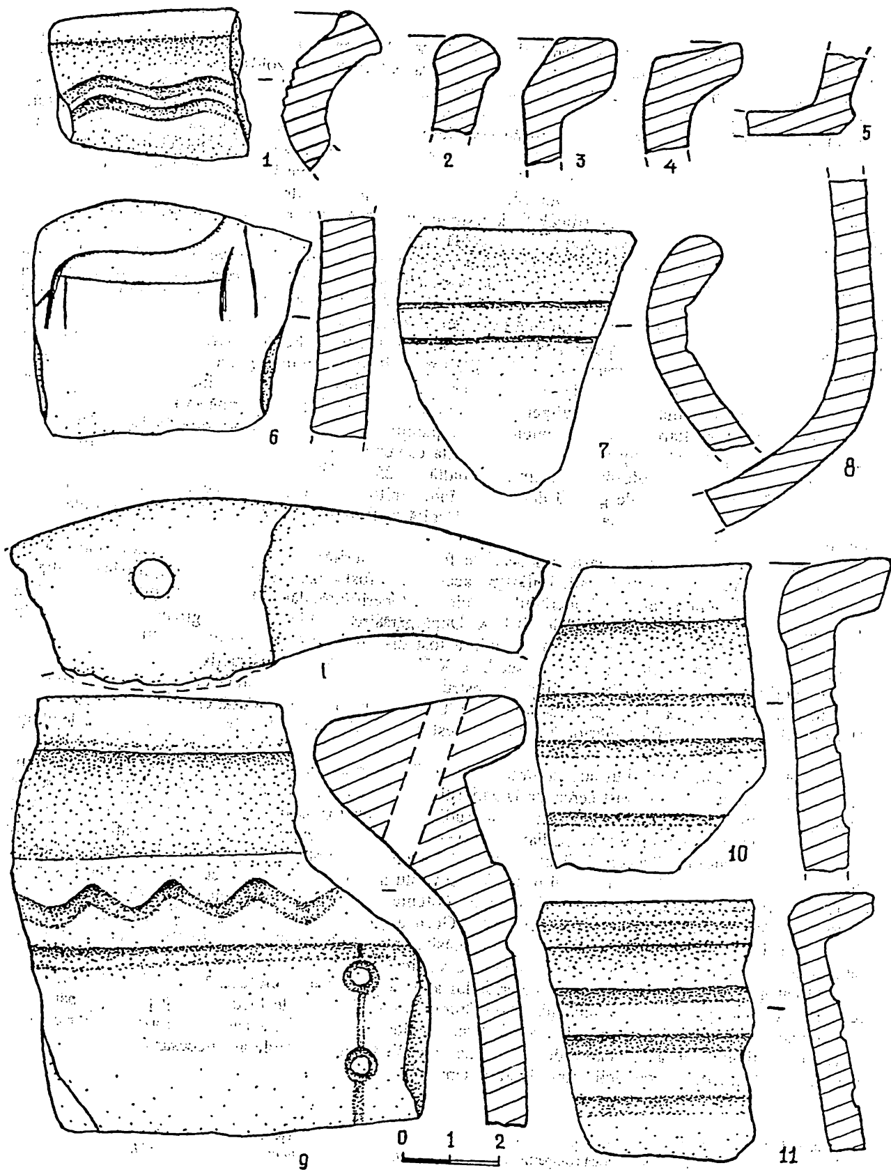
Fig. 9. Fragmente de oale-borcan (1, 7, 5) și de căldări de lut (2-4, 6, 8-11) din secolele XI-XII, descoperite în locuințele 16 (4-5, 7-8) și 24 (1-2), în cuptoarele 8 (6, 10) și 9 (3, 9) și în stratul cultural (11).
