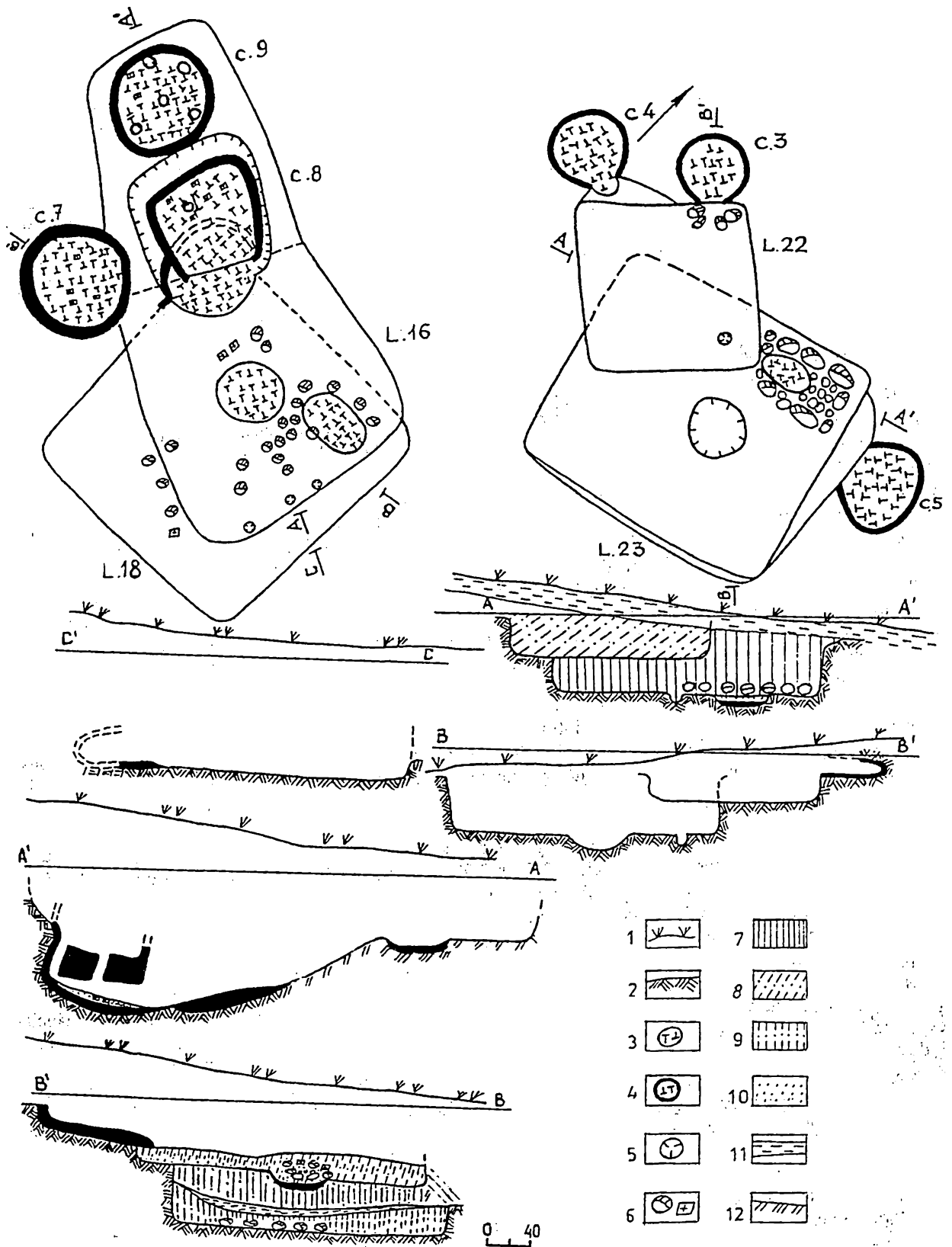
Fig. 3. Locuințele nr. 16, nr. 18, nr. 22, nr. 23, plan și profil, și cuptoarele de copt pâine nr. 3-5, și de ars ceramica – simple (nr. 7) și cu grătar (nr. 8 și nr. 9). 1, nivelul actual de călcare; 2, sol galben steril; 3, vatra cuptorului din piatră; 4, vatra cuptorului cotlonit; 5, gropi; 6, piatră, ceramică; 7, nivel de secolele VIII-X; 8, strat cu cenușă; 9, nivel cu căldări de lut; 10, cenușă; 11, sol vegetal; 12, strat cultural.
