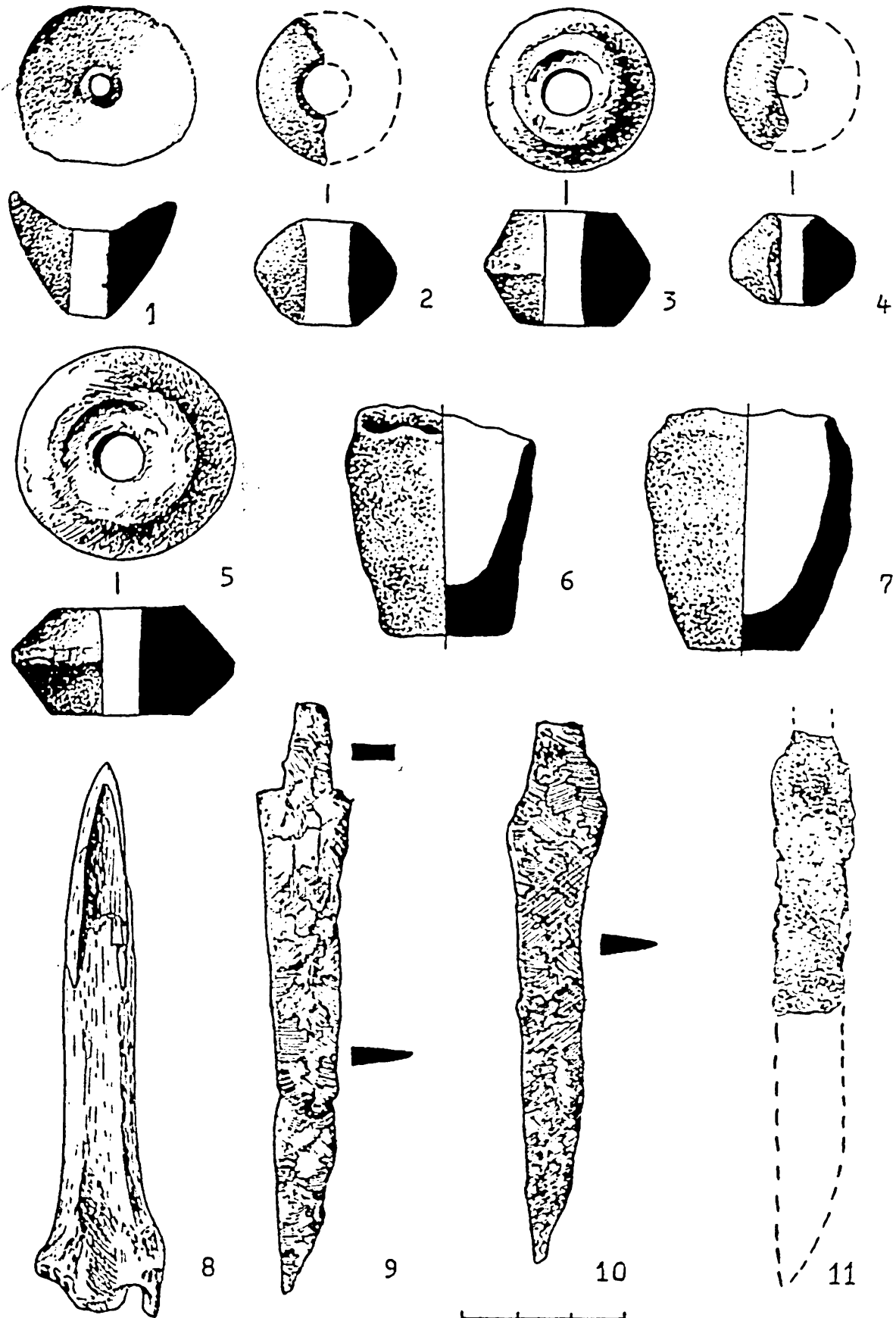
Fig. 4 Unelte din fier (9-11), lut (1-5) și os (8) și obiecte din lut (6-7) 5 - locuința 17; 3, 11 - locuința 22; 2, 4, 6-8 - locuința 25; 1, 9 - strat cultural
