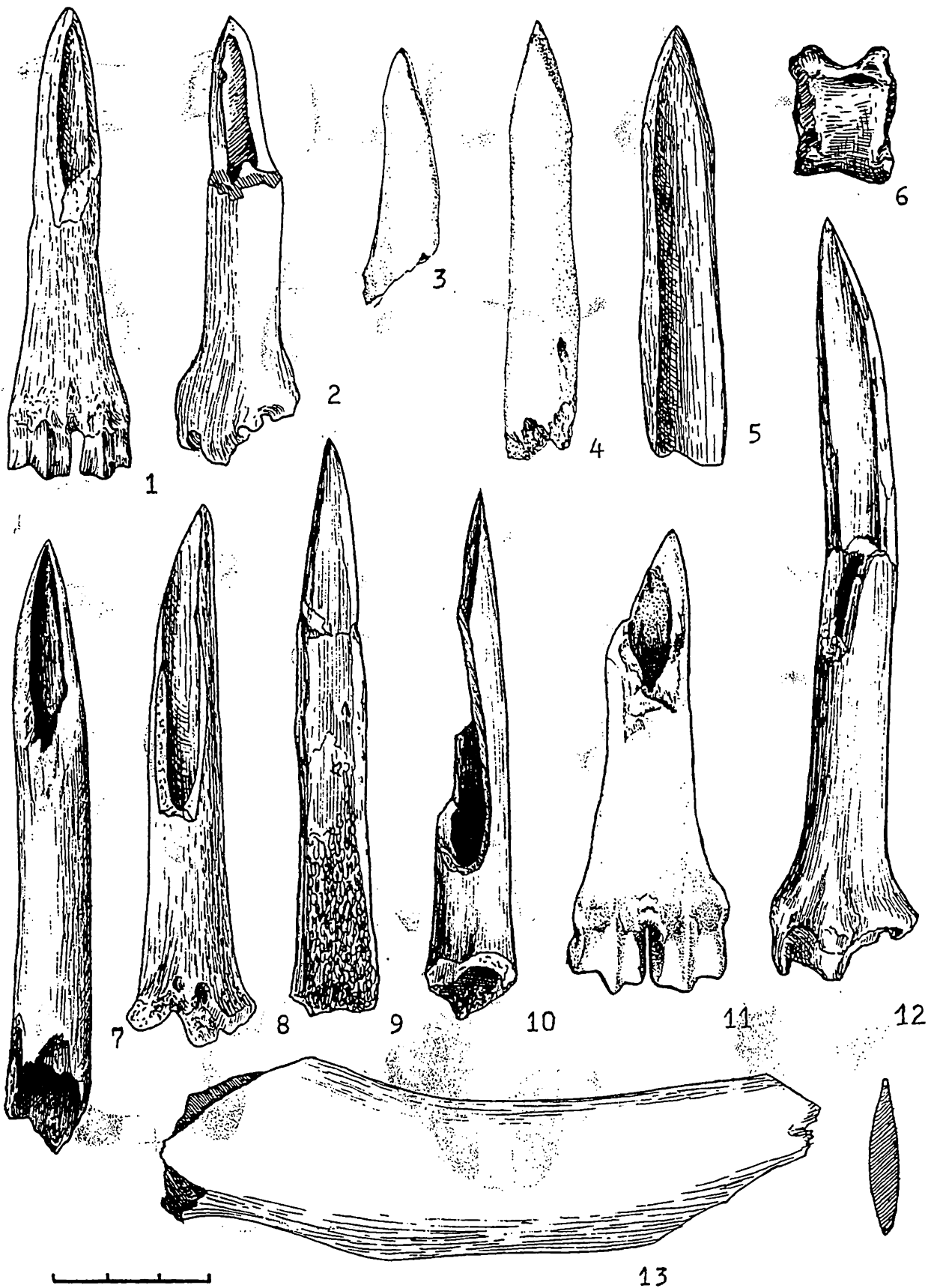
Fig. 6. Unelte și obiecte din os. 1-3, 13 – locuința 14; 7-10, 12 – locuința 17; 4-6 – locuința 22; 11 – locuința 23.
