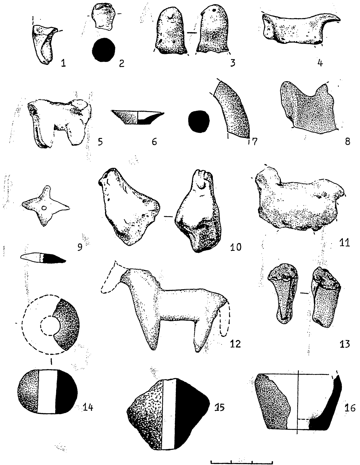
Fig. 7. Uñelte și obiecte din lut. 2-4 – locuința 14; 1, 6-8, 14 – locuința 23; 10, 16 – locuința 25; 5, 11-13 – strat cultural.
