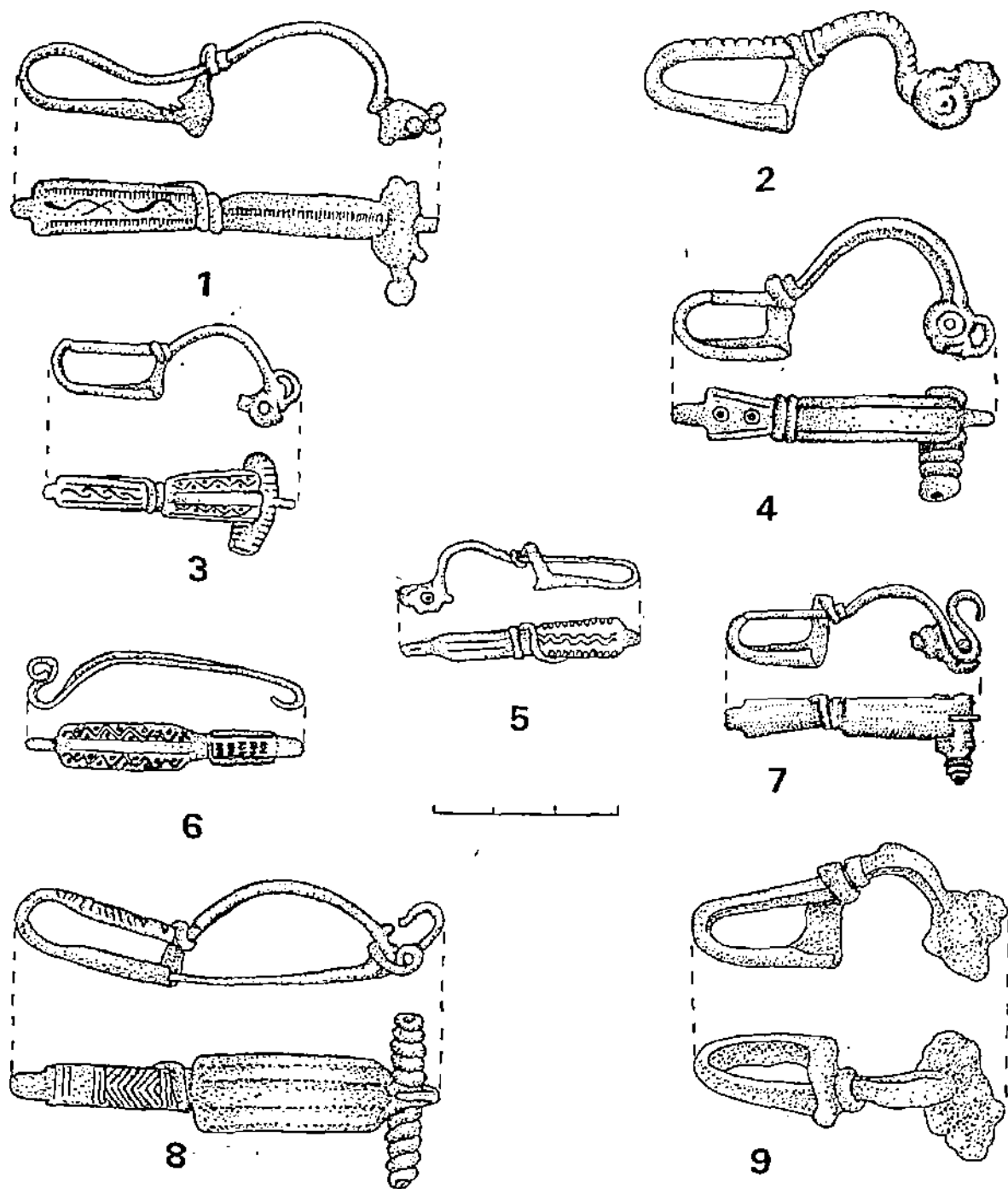
Fig. 3. Fibule din bronz cu piciorul înfășurat, din secolul al VI-lea e.n. 1,3-4, Cetei-Olt; 2, Budureasca-Prahoza; 5-6, București-Militari; 7-8, Localități necunoscute (Muntenia, Oltenia ?); 9, Tîrșoru Vechi-Prahoza.
