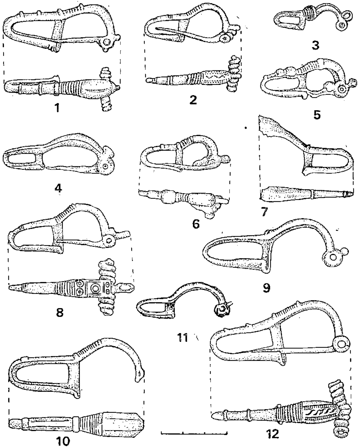
Fig. 7. Fibule din bronz turnate, din secolele VI–VII e.n. 1–2, 8, 12, Localități necunoscute (Muntenia, Oltenia ?); 3–6, 9–11, Cei–Olt; 7, Tîrșoru Vechi–Prahova.
