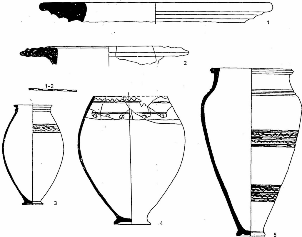
Fig. 3. Vase cu buza orizontală, lată (1, Costești-Cetățuic; 2, Căpâlna) și cu ornamente diferite (3, 5 Răcățu; 4, Grădiștea de Munte-Meleia).
