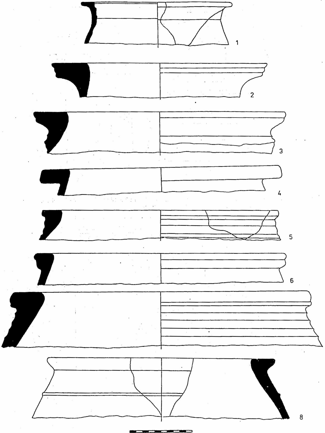
Fig. 1. Vase cu buza orizontală, îngroșată (1, Căpâlna; 2-8, Costești-Cetățuic).
