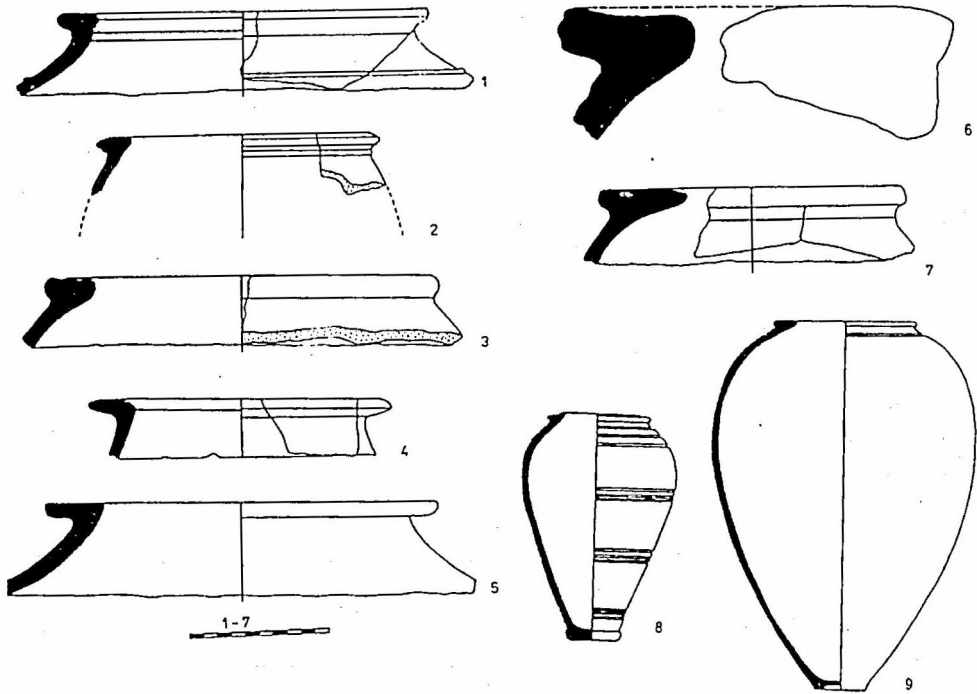
Fig. 2. Vase cu buza orizontală, trasă spre interior (1, 4, 6-7, Căpâlna; 2-3, Divici; 5, Costești-Cetățuic; 8, Izbiște; 9, Costești-Blidaru).
