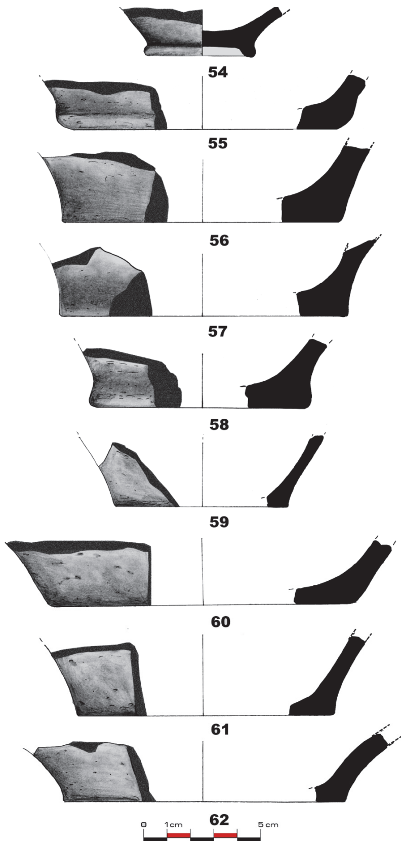
Pl. XI. Gănești - Tironu . Funduri de vase (54-62).
