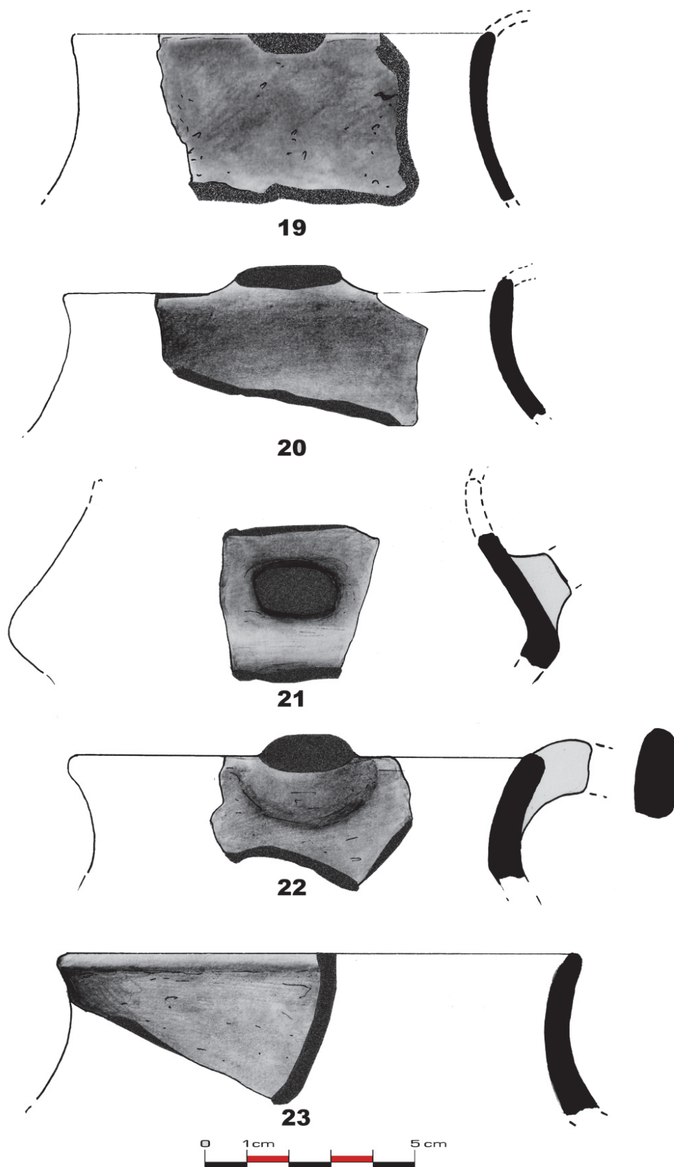
Pl. VI. Gănești - Tironu. Căni (19-23).
