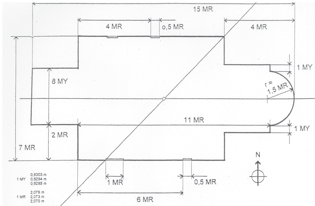
Abb. 2 Grundriss der Wormbacher Pfarrkirche in den megalithischen Masseinheiten MY und MR.
