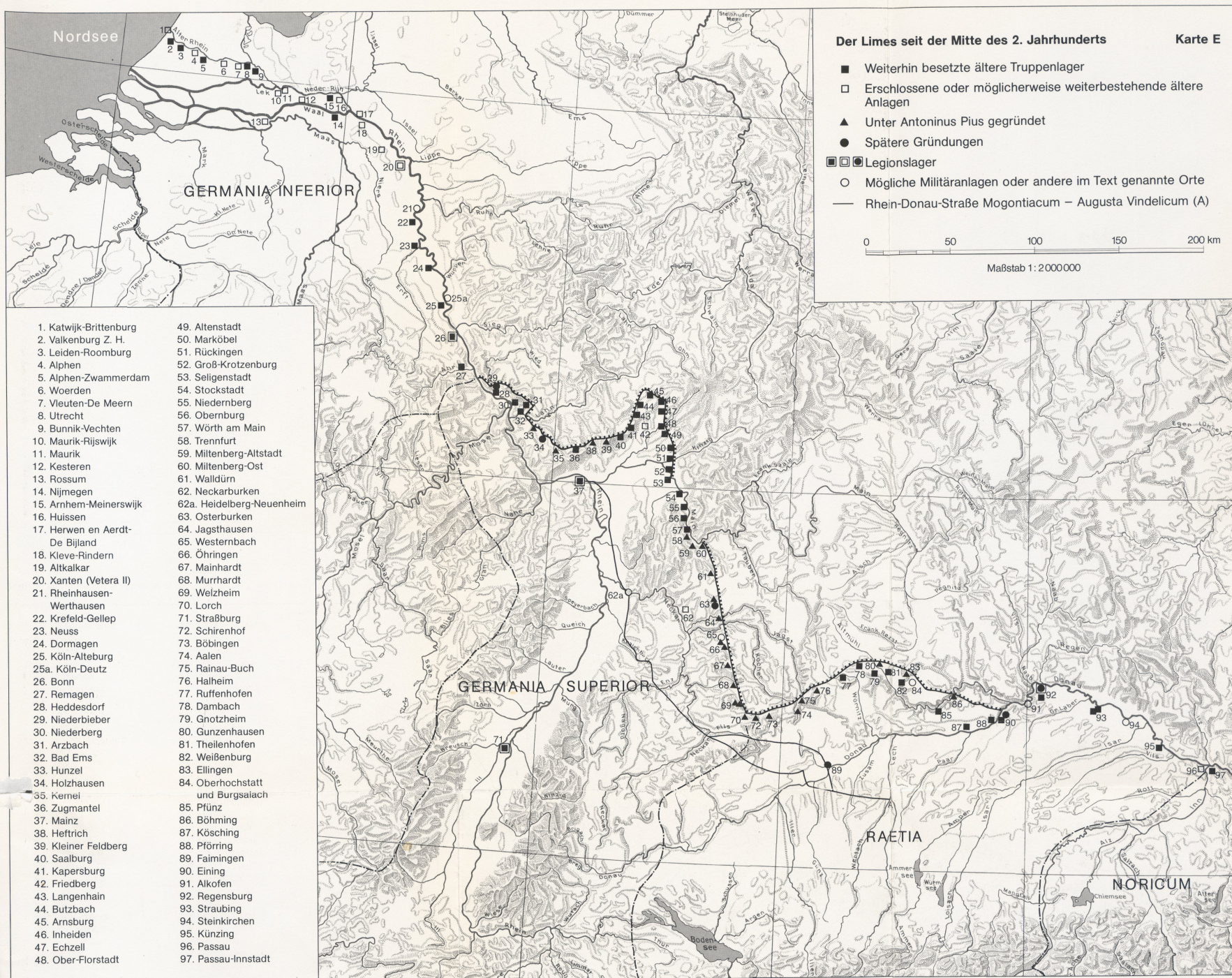
Karte E: Der Limes seit der Mitte des 2. Jahrhunderts. M. 1:2 000 000.
