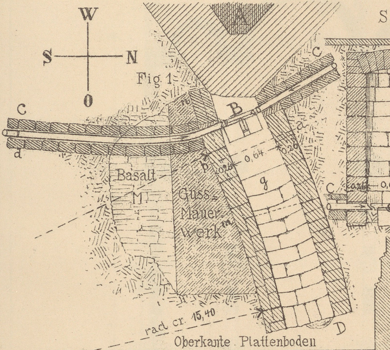
Grundriss
