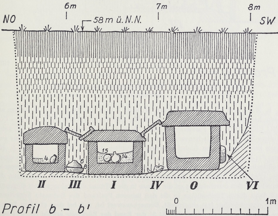
Abb. 7. Querschnitt b-b' durch die Gräbergruppe (siehe Abb. 4-5). Maßstab 1 : 25.
