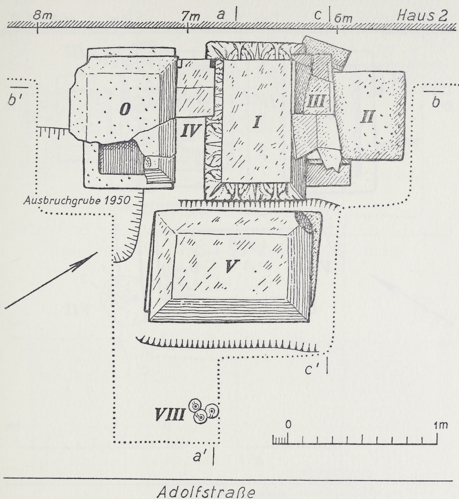
Abb. 4. Gräbergruppe an der Adolfstraße im Zustand der Auffindung. Maßstab 1 : 25.
