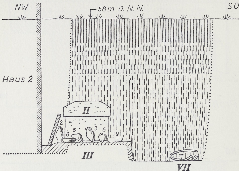
Profil c - c'
