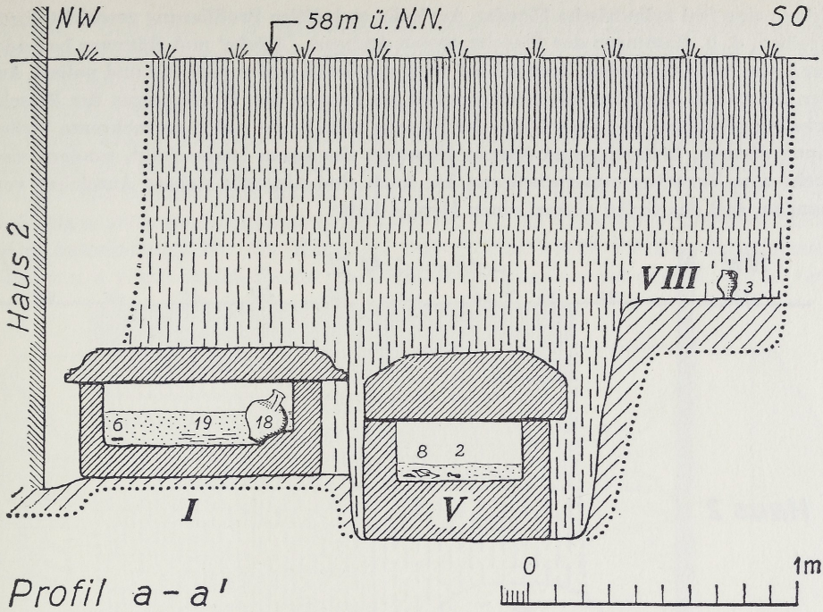
Abb. 6. Querschnitt a-a' durch die Gräbergruppe (siehe Abb. 4-5). Maßstab 1 : 25.
