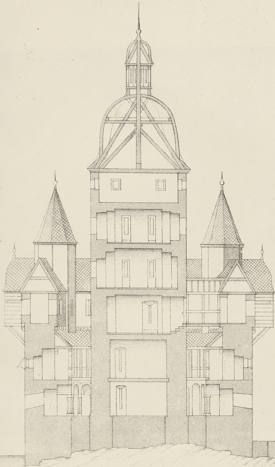
Querschnitt.
