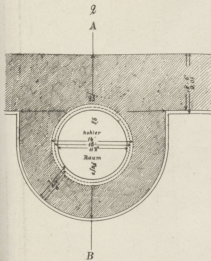
Grundriß von Thurm XIII mit dem Sockel
