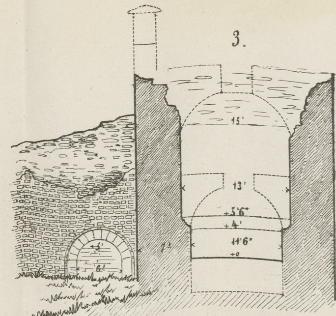
Ansicht der Pforte und Durchschnitt durch die Mitte des Thurms VI in der Richtung der Mauer.
