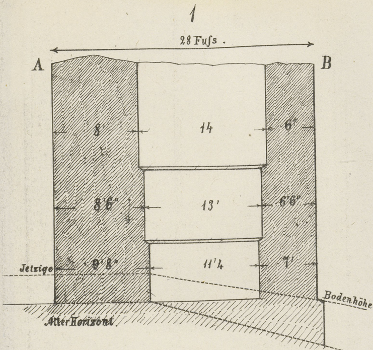
Durchschnitt von Thurm XIII quer durch die Mauer.
