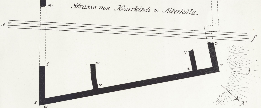
Grundriss unterhalb des Fussbodens.
