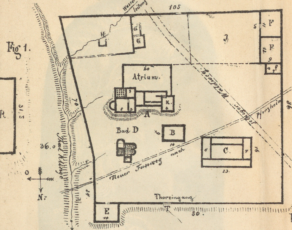
Wohnhaus der Villa im Sinzheimer Wald 1:400
