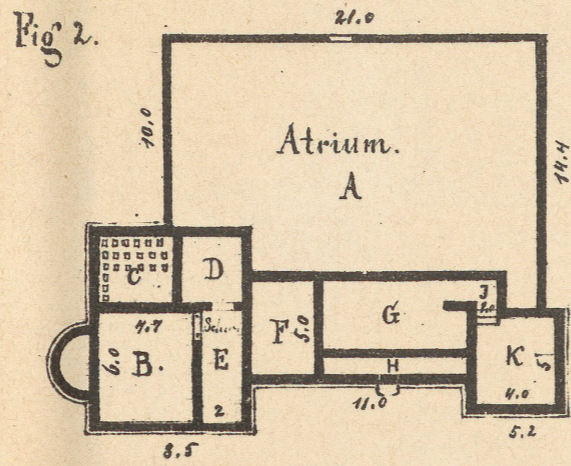
Thür- und Thorschwellen in A u. E.
