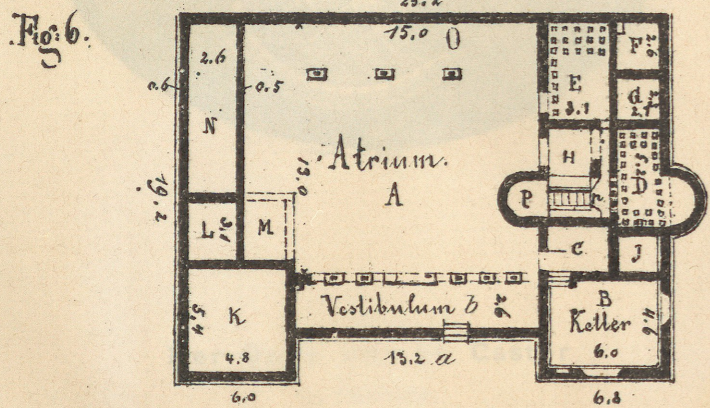
Wohnhaus der Villa im Sinzheimer Wald 1:400
