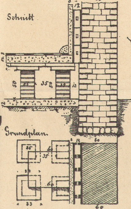
Fig. 12 Hypocaustum. 1:40.
