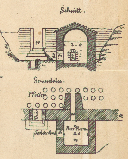
Fig. 13. Praefurnium in Baden.
