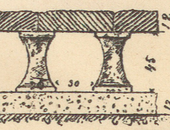
Steinleiter. 1:40.
