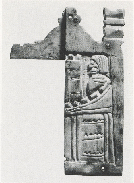
1a–b Spiegelfassung (Fragment) aus Knochenstreifen von Burg Hain (Dreieichenhain, Hessen). Innen- und Außenseite. Museum Dreieich. – Maßstab 1:1.
