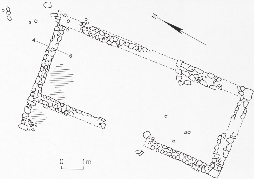
3 Abenden, Matronenheiligtum. Gebäude I. – Maßstab 1 : 100.
