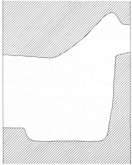
6 Mithrasstein aus Bonn. Schnitt durch die Beleuchtungsvorrichtung. – Maßstab 1 : 3.
