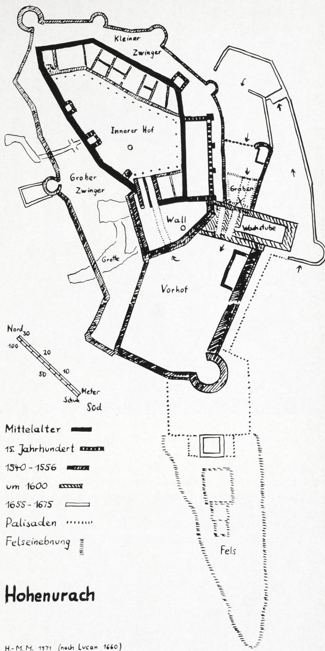
Abb. 3. Grundriß der Festung Hohenurach mit einer Übersicht über die einzelnen Bauepochen
