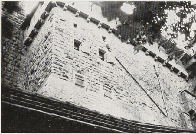
Abb. 4. Nordostecke der Kernburg von Nordosten; links die Fuge zwischen Bergfried und östlicher Ringmauer, rechts der Eckverband (?) zwischen dem höheren Buckelquaderbauteil an der Ecke (von Ebhardt restauriert) und dem niedrigeren (Ringmauer) an der Nordseite (Foto Th. Biller)
