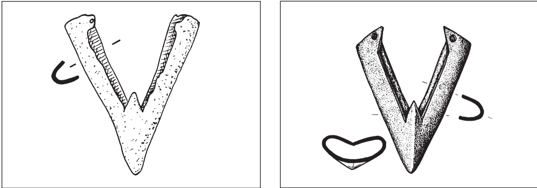
Abb. 5 (links): Ortband von der Kronenburg bei Dossenheim a. d. Bergstrasse. M 1 : 2. – Abb. 6 (rechts): Ortband aus Braunschweig. M 1 : 2.
