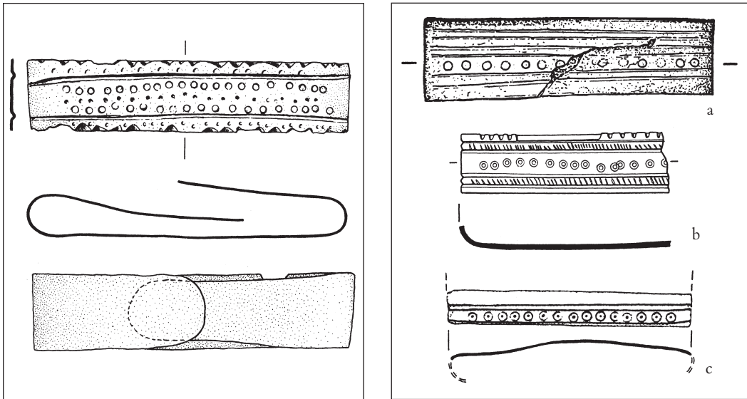
Abb. 1 (links): Scheidenmundblech aus Tauberbischofsheim. M 2:3. – Abb. 2 (rechts): Scheidenmundbleche mit schlichtem Rillen- und Kreiskekor aus Heidenheim-Großkuchen (a), Frankfurt-Praunheim ‚Ebel‘ (b) und vom Runden Berg bei Urach (c). M 2:3.
