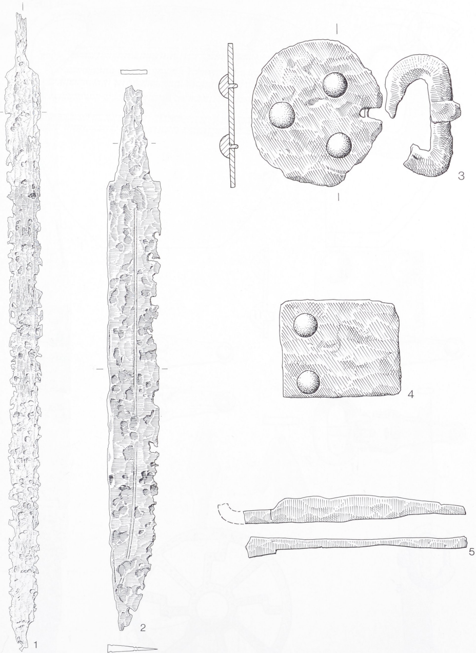
Abb. 7 Iffezheim, Grab 2. M 1:2, außer 1 M 1:5 und 2 M 1:3.
