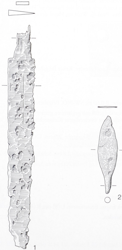
Abb. 6 Iffezheim, Grab 1. M 1:2.
