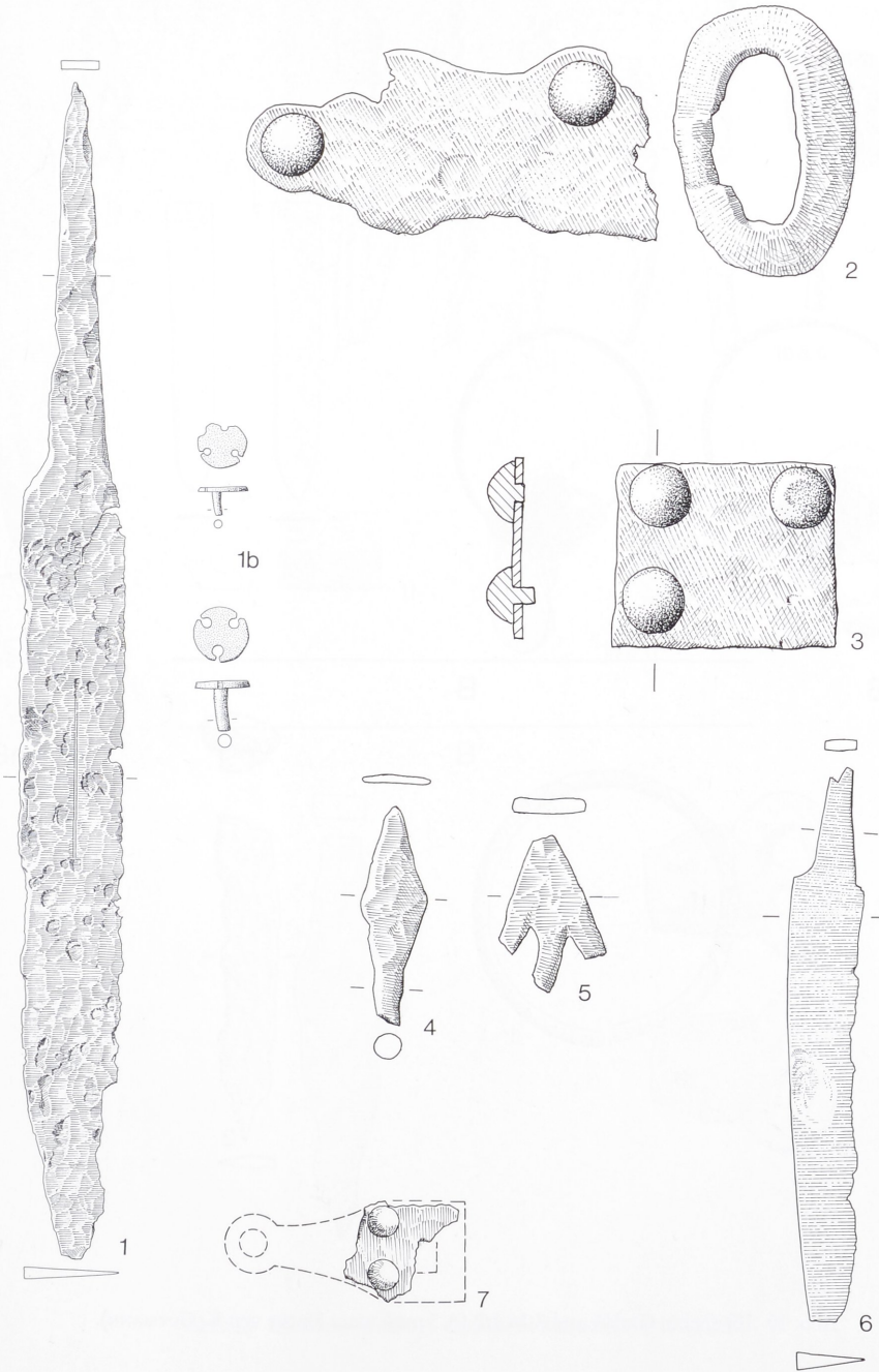
Abb. 9 Iffezheim, Grab 4. M 1:2, außer 1 M 1:4.
