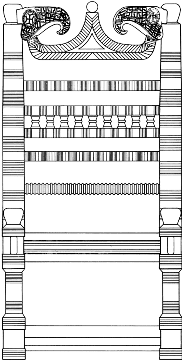
13 Oberflacht Grab 11. Rekonstruktion der Rückenlehne des Stuhles mit den Tierköpfen (ohne Maßstab).
