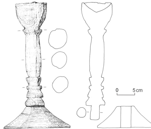
5 Trossingen Grab 58. Der Eichenleuchter.
