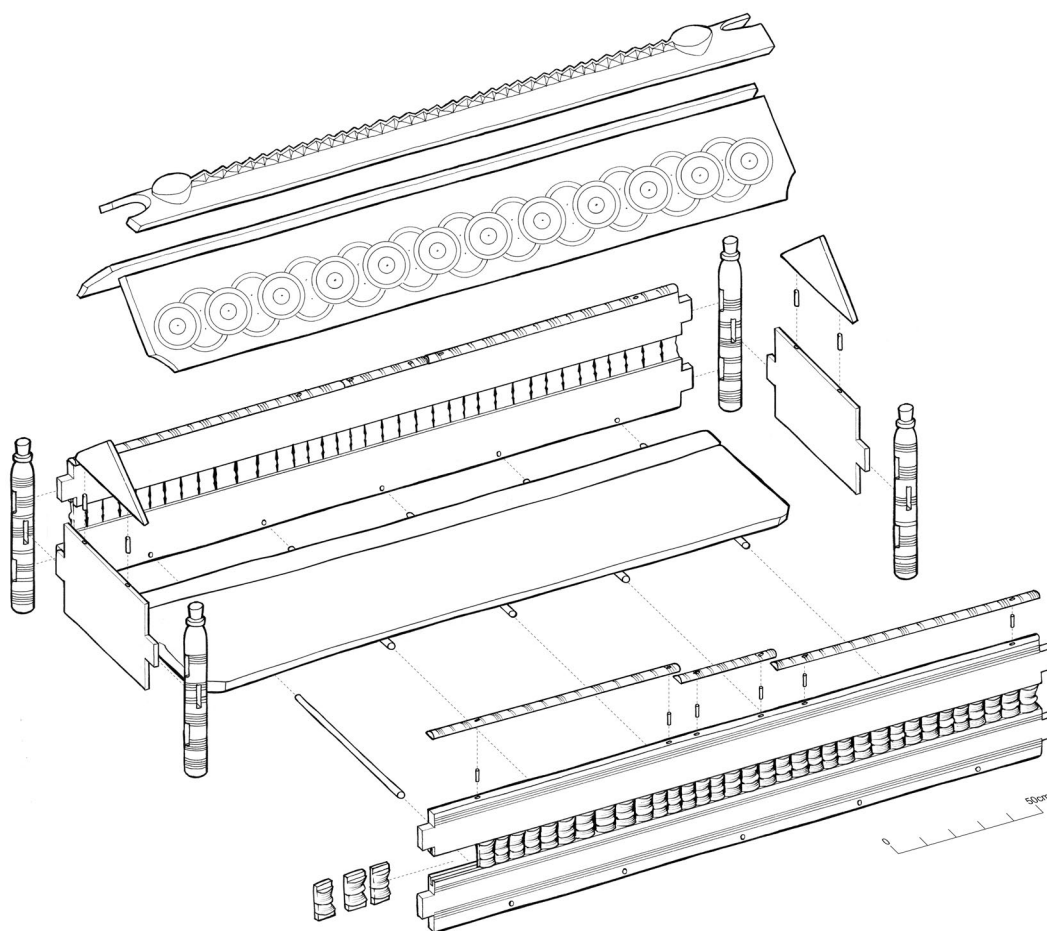
4 Trossingen Grab 58. Konstruktionsdetails von Rahmenbett und Dachaufsatz.
