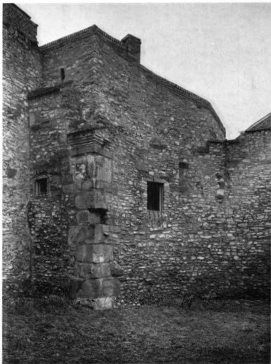
Abb. 1: Erhaltene Südostecke der Aula Regia in Ingelheim mit Ansatz der Apsis
