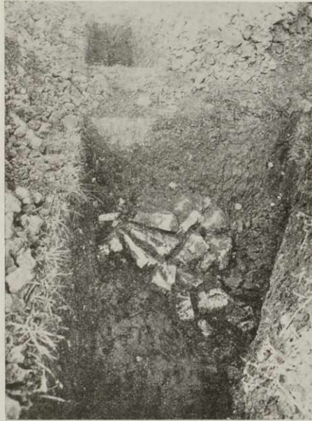
Abb. 3. Schnitt 13 von Südosten: Unten die natürliche Lehmaböschung, darüber die künstliche Steinböschung.
