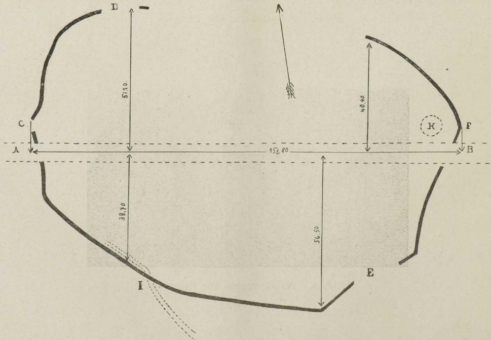
Abb. 2. Mauerring am Südosthang des großen Feldbergs. 1 : 1350.
