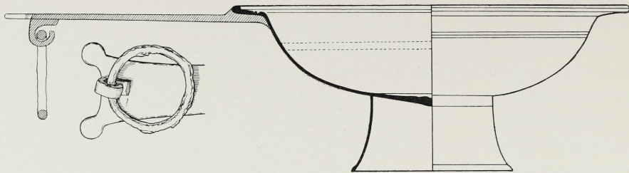
Abb. 2. Pfanne von Güttingen. Längsschnitt und Griffende von unten. 1:3.
