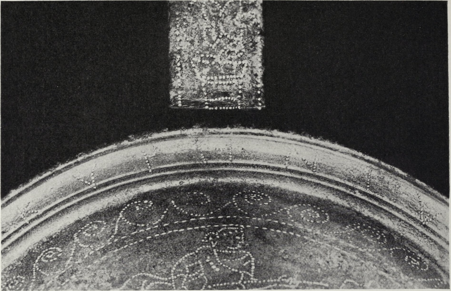
Abb. 4. Pfanne von Göttingen. Teilansicht von Griff und Schale. Etwa 1:1.
