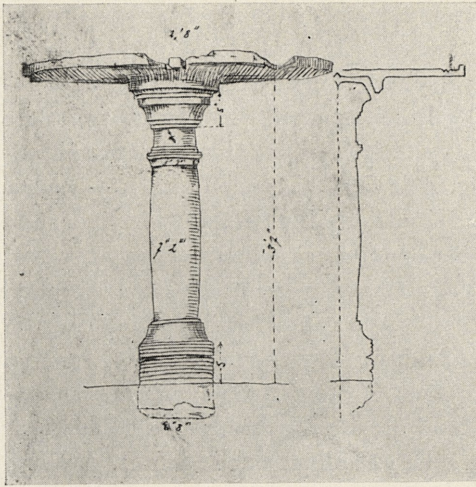
Abb. 4. Tisch aus dem Tempel bei Bretten (Baden). M. 1:30.
