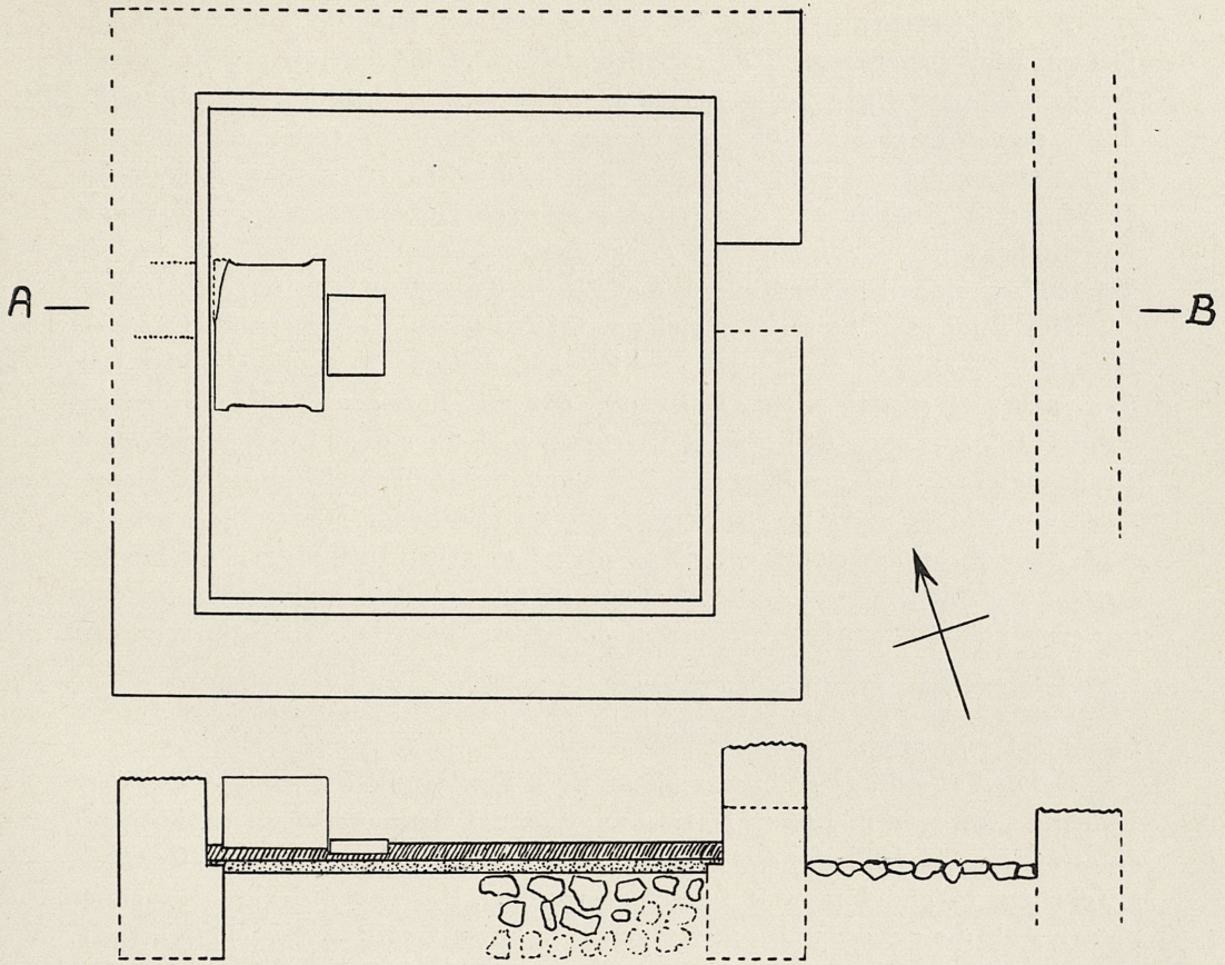
Abb. 1. Plan und Schnitt des gallo-römischen Tempels bei Bretten (Baden) M. 1:60.
