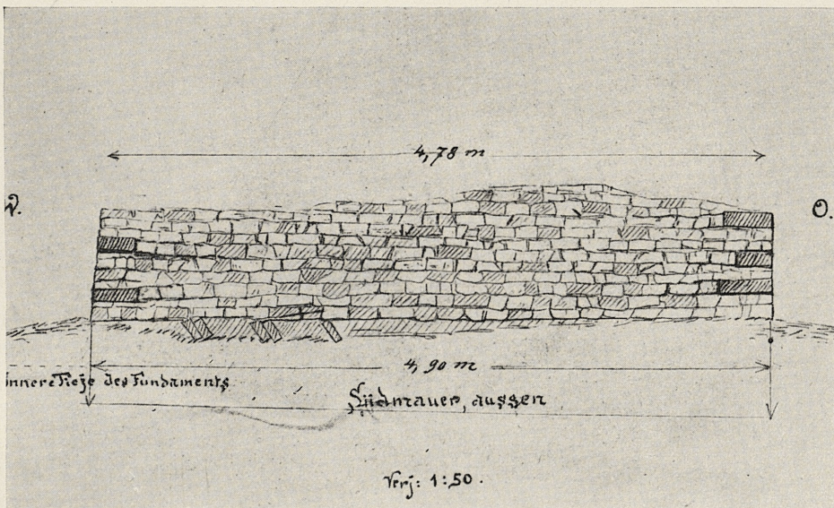
Abb. 2. Südmauer des Tempels bei Bretten (Baden). M. 1:50. (Zeichnung Wörners.)
