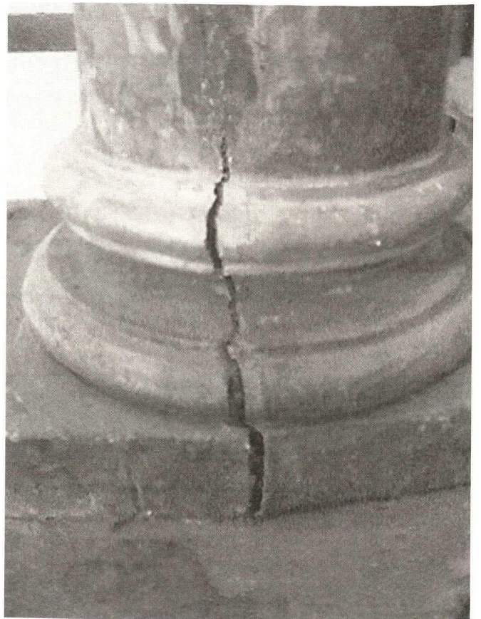
Grietas en estructura por cambios de humedad
