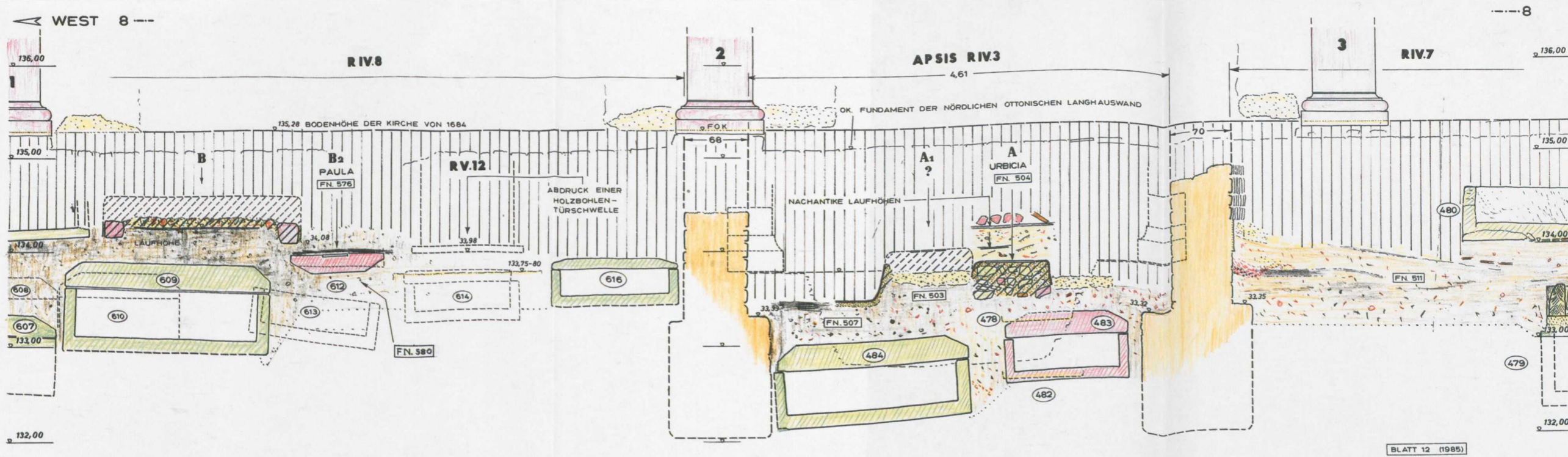
Trier, St. Maximin. – Oben: Nord-Süd-Schnitt 134-134 durch den Apsidenraum R IV. 3 mit der VRBICIA-Inschrift A. – Unten: West-Ost-Schnitt 8-8 im nördlichen Seitenschiff der Kirche, durch die gemauerte Inschriftfassung und Grabschrift der VRBICIA A sowie durch das Blockmauerwerk B im Raum R IV. 8 über dem Grab 609; Schnitt durch den Grabstein der PAVLA B2 (mit Inschrift). – M = 1:50.
