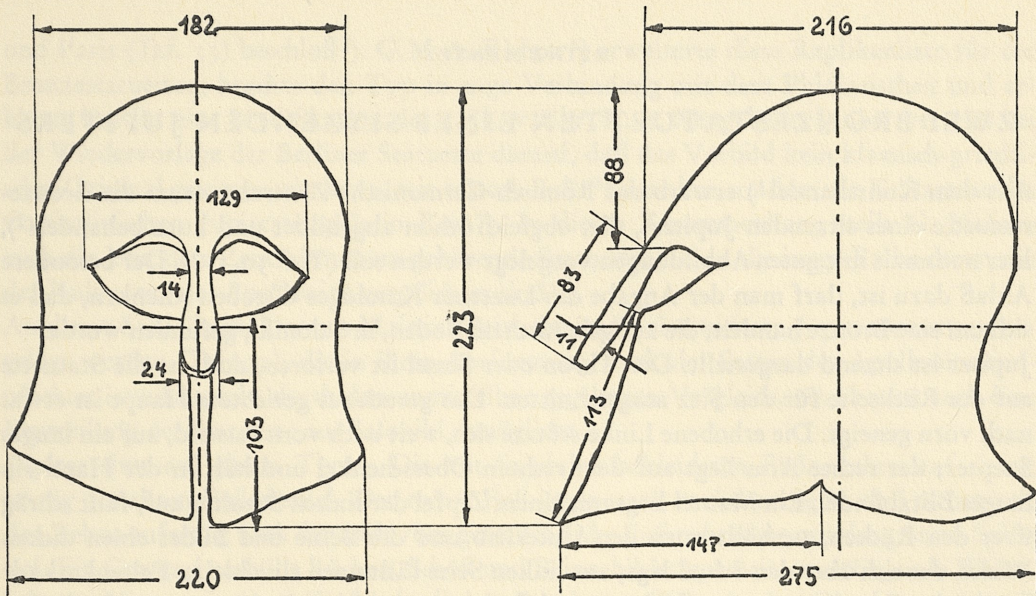
Abb. 1 Maße des Helmes
