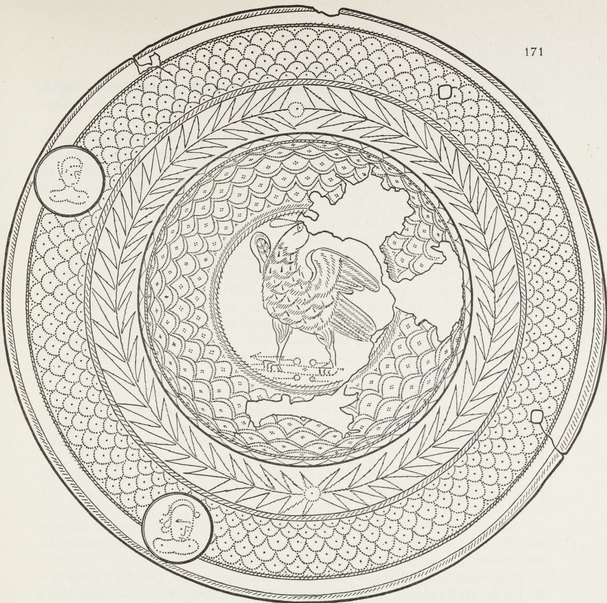
Abb. 3 Bronzeschildbuckel B. Fo. Mainz. Mus. Wiesbaden. M = 3:4.
