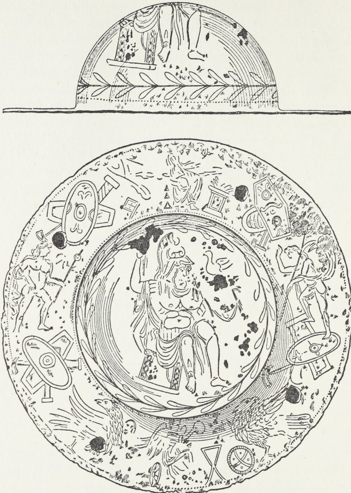
Abb. 11 Bronzeschildbuckel. Fo. Kirkham. Brit. Mus. London. M. = 1 : 2.
