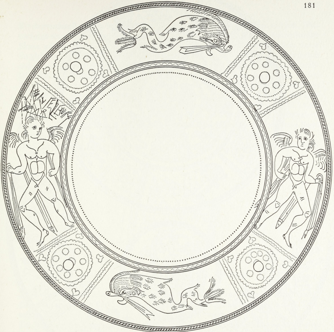
Abb. 7 Bronzeschildbuckel. Fo. Hälmeag. Mus. Sibiu. Verzierung des Randes. M. = 3 : 4.
