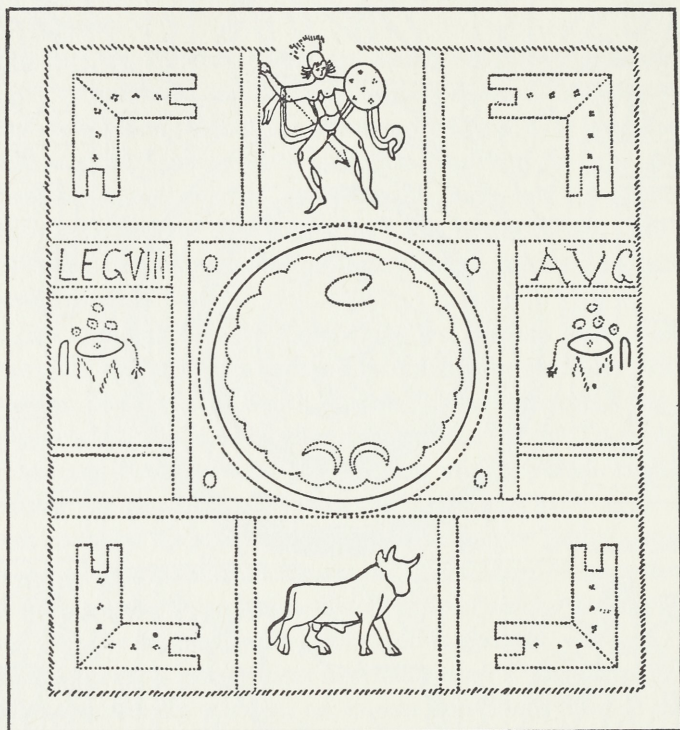
Abb. 6 Bronzeschildbuckel. Fo. Windisch. Vindonissamus. Brugg. Rekonstruktion (nach Ch. Simonett). M = 1:3.
