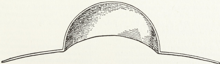
Abb. 5 Bronzeschildbuckel. Aus dem Tynefluß bei South Shields. Brit. Mus. London. M = 1:2.
