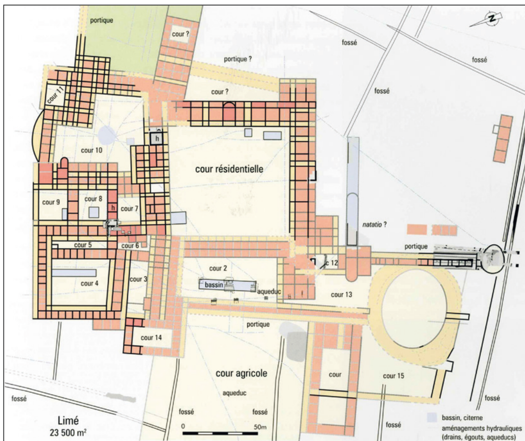
Fig. 25 La partie résidentielle de la villa de Limé (départ. Aisne/F). – (D’après Collart 2013, 105).
