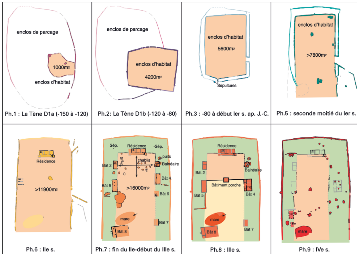
Fig. 8 Évolution chronologique de la villa de Roye (dép. Somme/F). – (D'après Collart 2013, 96).
