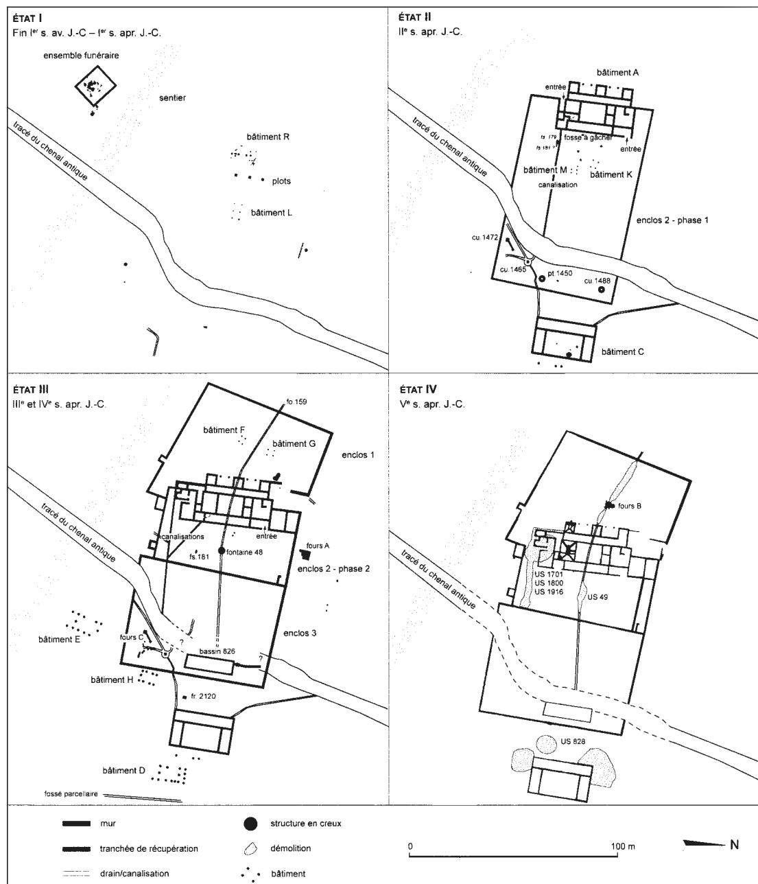
Fig. 19 Développement de la villa de Grigy (départ. Moselle/F). – (D'après Brkojewitsch et al. 2014, fig. 3).
