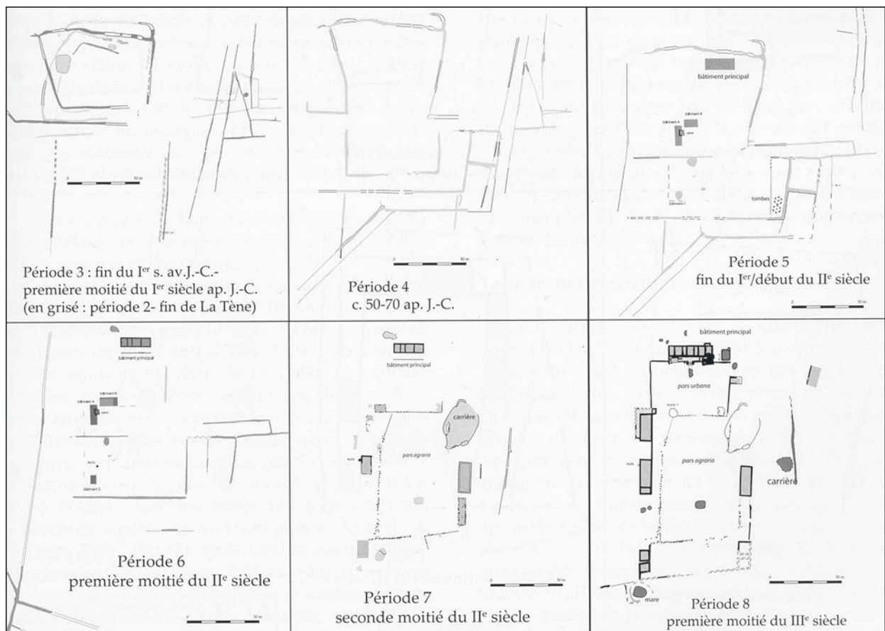
Fig. 9 Évolution chronologique de la villa de Behen (dép. Somme/F). – (D'après Bayard/Lemaire 2014, fig. 68).
