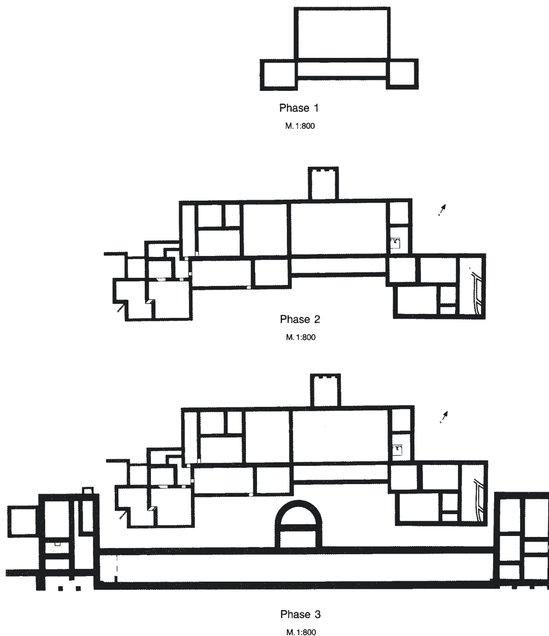
Fig. 20 Développement chronologique de la villa de Leudersdorf »Bannweiler« (Lkr. Vulkaneifel/D), dans l'Eifel. – (D'après Henrich 2006, pl. 55).
