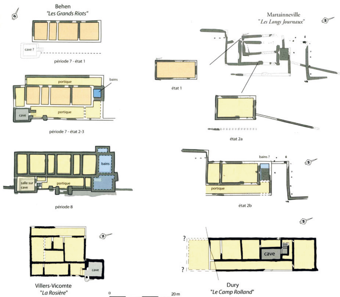
Fig. 16 Plans des résidences principales de Behen (départ. Somme/F), Martainneville (départ. Somme/F) et Villers-Vicomte (départ. Oise/F), Dury (départ. Somme/F). – (D'après Bayard/Lemaire 2014, fig. 73).
