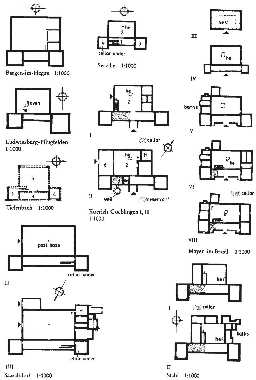
Fig. 18 Hall houses. – (D'après Smith 1997, 25).
