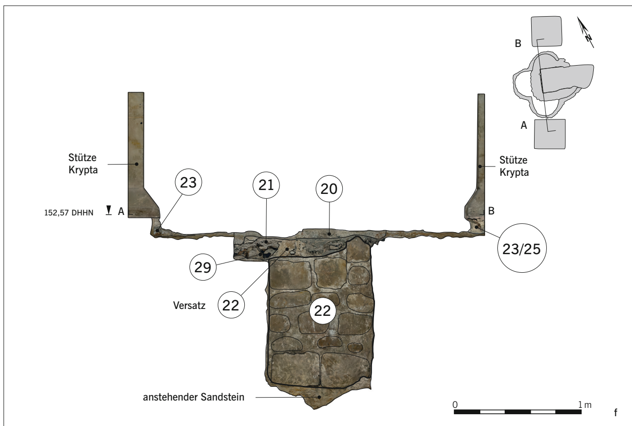
Abb. 9e–f Quedlinburg, Krypta St. Servatii. A 17364: Die Befunde. Verzerrungsfreie Orthobilder in Richtung SSW (e) und WNW (f) nach Abnahme von Steinen aus der obersten Reihe des gemauerten Schachtes (Befund 22) im Süden und Westen sowie partielle Freilegung der Auskleidung des Vierpasses (Befund 20) im Süden (vgl. Abb. 8b; 12).
