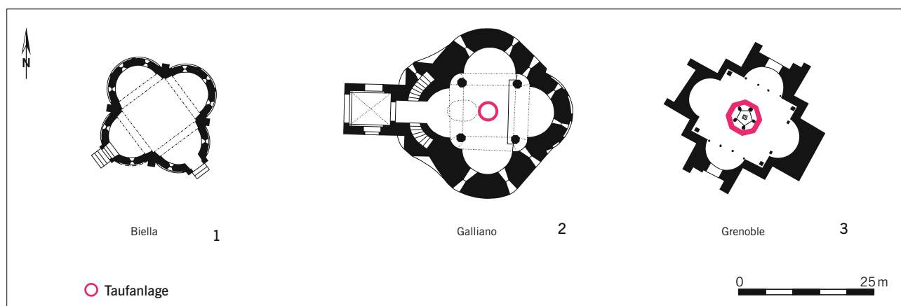
Abb. 24 Vierpassförmige Grundrisse von Baptisterien aus dem 10. Jh. und dem Beginn des 11. Jhs.: 1 Biella, Piemont (IT); 2 Galliano, Lombardei (IT); 3 Grenoble, Dép. Isère (FR).
