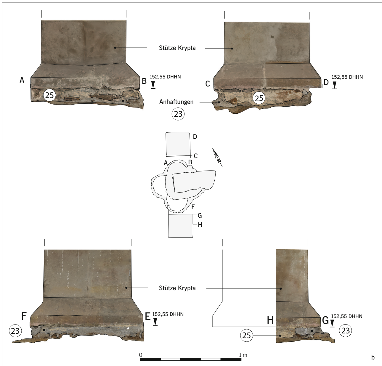
Abb. 9b Quedlinburg. Krypta St. Servatii. A 17364: Die Befunde. Profile an den Kryptastützen.
