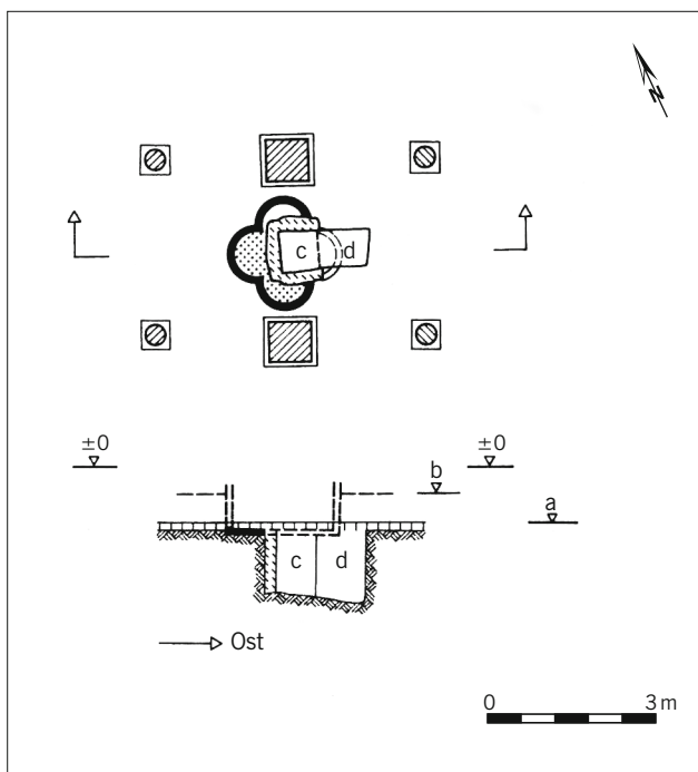
Abb. 6a–b Quedlinburg, Krypta St. Servatii. Die Vierpassstruktur wurde bereits in den 1930er-Jahren durch den Ausgräber Hermann Wäscher erfasst. Sie wurde bei den aktuellen Ausgrabungen gezielt wieder aufgedeckt und so vorgefunden, wie von ihm durch insgesamt zwei mäßig instruktive Fotos dokumentiert.
