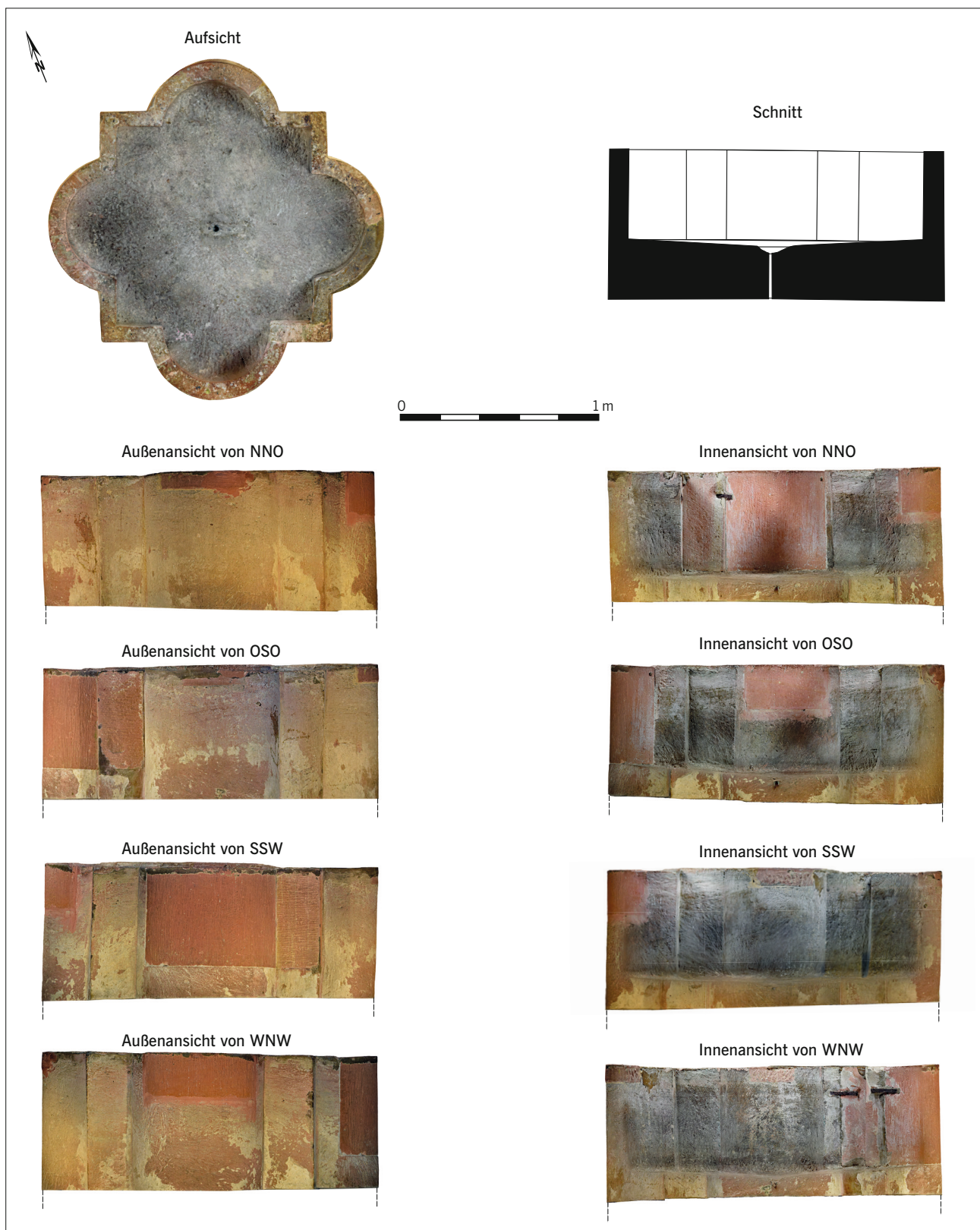
Abb. 23b Das Taufbecken aus der Krypta im Dom zu Speyer. Orthofotos.
