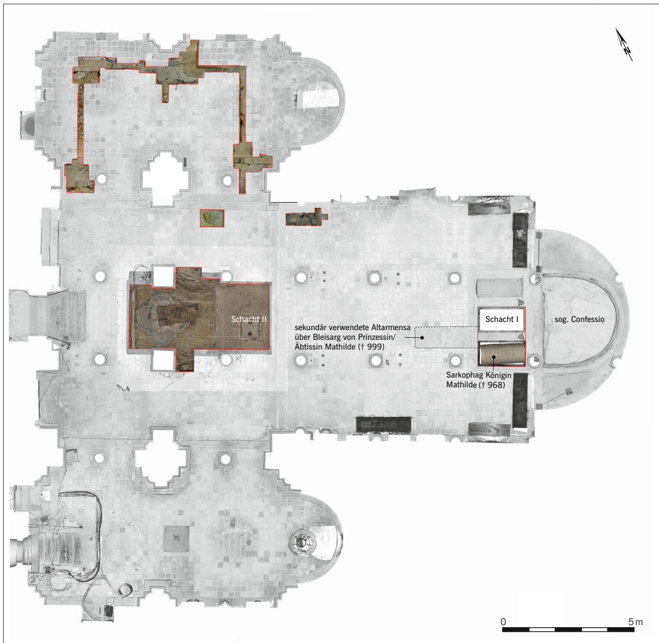
Abb. 4 Untersuchungsflächen 2023/24 (rot umrandet) in der Krypta der Stiftskirche St. Servatii zu Quedlinburg. Der Sarkophag der Königin Mathilde († 968) wurde nicht geöffnet.
