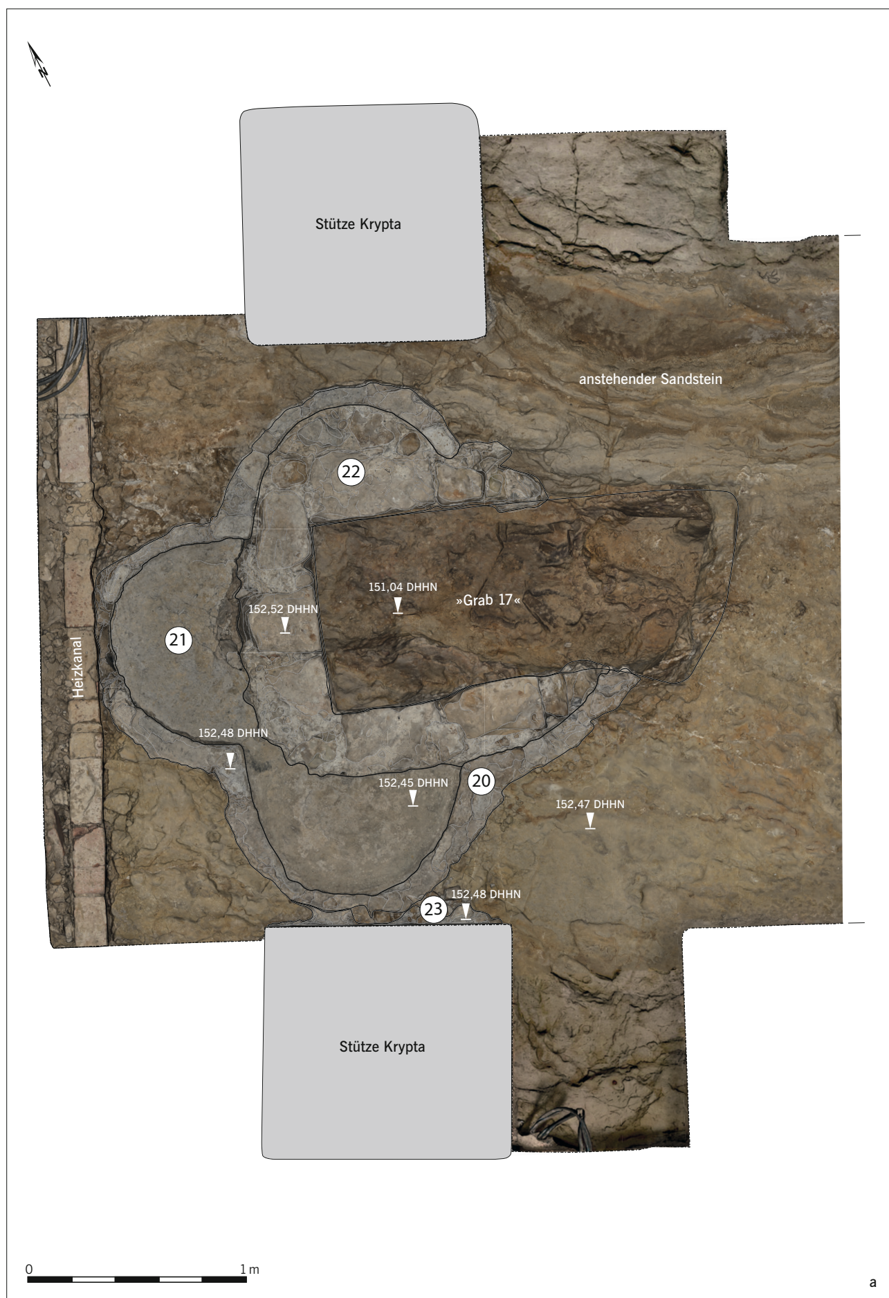
Abb. 9a Quedlinburg, Krypta St. Servatii. A 17364: Die Befunde. Aufsicht nach Absaugen der Sandverfüllung aus den 1930er-Jahren (vgl. Abb. 6a).
