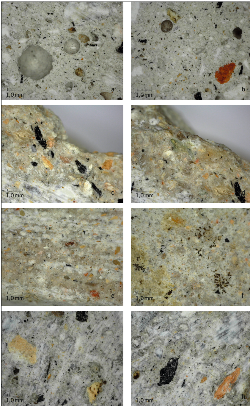
Abb. 11a–h Quedlinburg. Krypta St. Servatii. A 17364: Querschnitte von Gipsmörtelproben. a–b sekundär verbaute Estrichtrümmer Vierpass, Phase 1, Befund 20; c–d Versatzmörtel der Estrichtrümmer Wandung Vierpass, Phase 1, Befund 20; e–f Putzglätte/Ausgleichsmörtel Wandung Vierpass, Phase 1, Befund 20; g–h Estrichverguss Vierpass, Phase 2, Befund 21.
