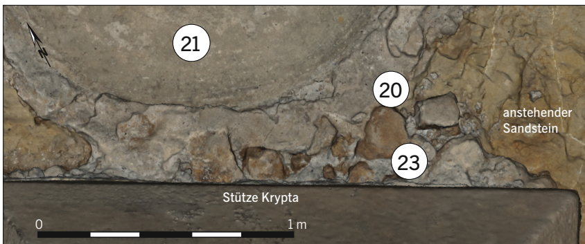
Abb. 16 Quedlinburg. Krypta St. Servatii. A 17364: Der Fußbodenestrich, Befund 23, verfügt über eine Steinstickung als Unterbau, die bis an den Vierpass zieht und diesen respek- tiert. Die in die Stickung geflossenen Estrich- spuren ziehen ebenfalls nicht über den Vier- pass, was darauf verweist, dass der Fußboden den Vierpass nicht überlagert.
