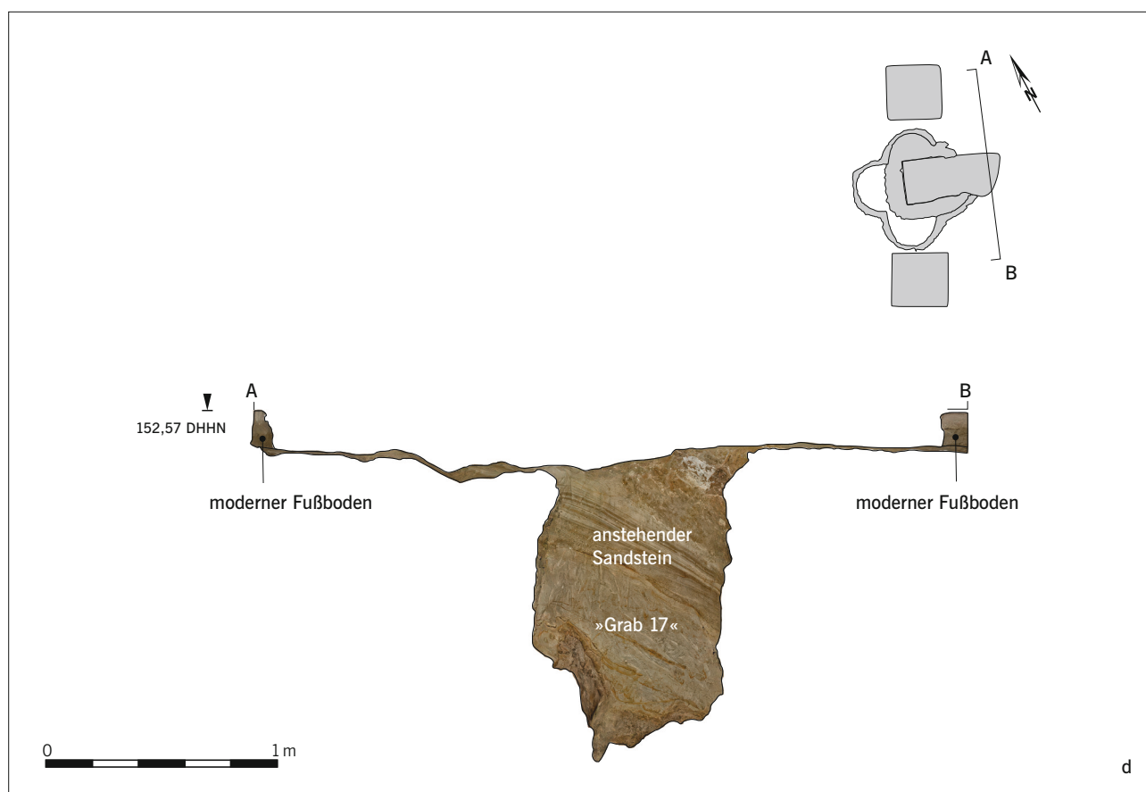
Abb. 9c–d Quedlinburg, Krypta St. Servatii. A 17364: Die Befunde. Verzerrungsfreie Orthobilder in Richtung NNO (c) und OSO (d) nach Abnahme von Steinen aus der obersten Reihe des gemauerten Schachtes (Befund 22) im Süden und Westen sowie partielle Freilegung der Auskleidung des Vierpasses (Befund 20) im Süden (vgl. Abb. 8b; 12).
