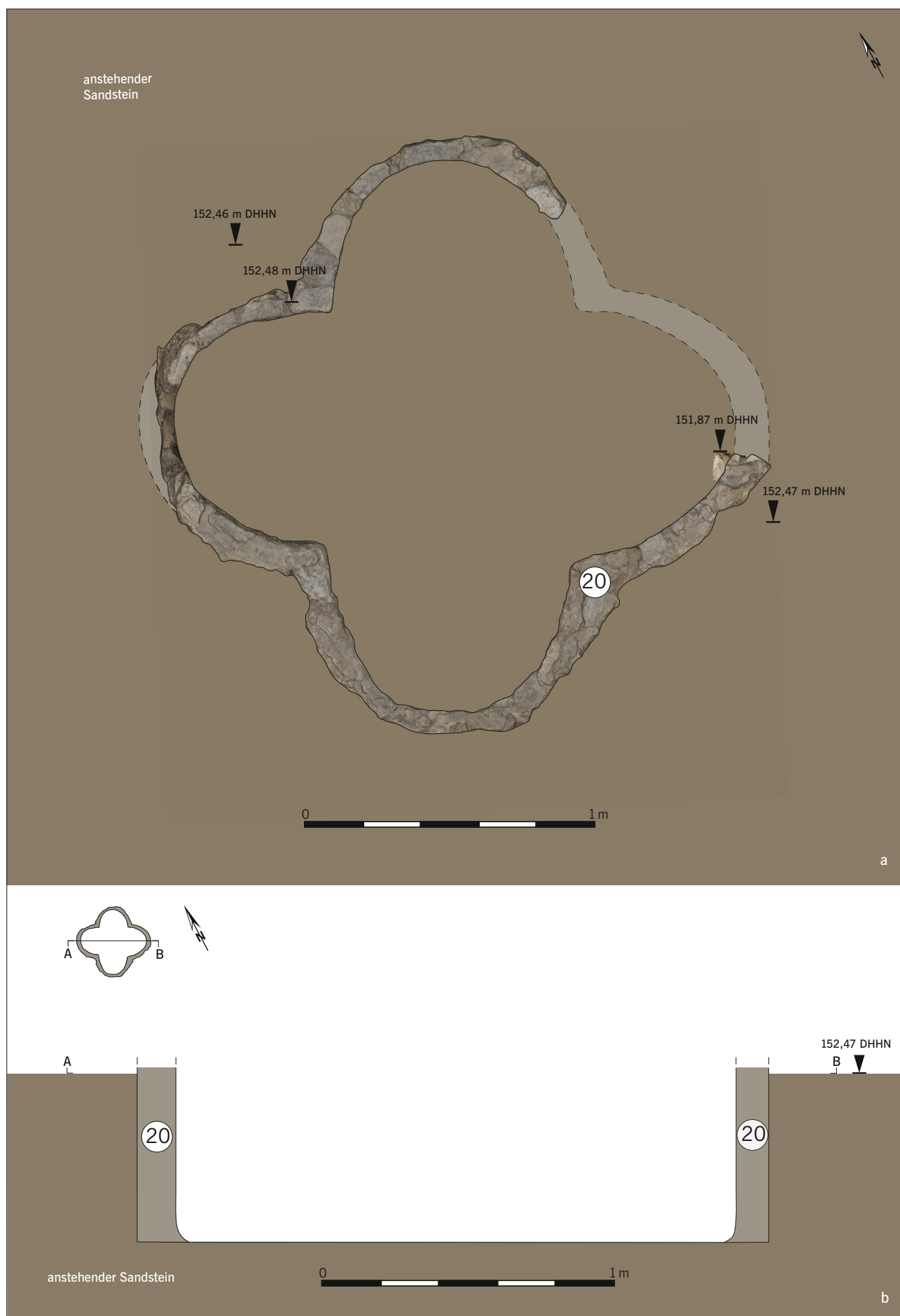
Abb. 10a–b Quedlinburg. Krypta St. Servatii. A 17364: Die Befunde der Phase 1. a Aufsicht; b schematischer Schnitt.
