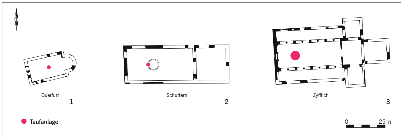
Abb. 18 In der Ottonenzeit wurden Taufanlagen üblicherweise auf die Mittelachse des Langhauses gesetzt. Archäologisch erfasste Taufanlagen: 1 Burgkirche von Querfurt, Saalekreis, zweite Hälfte 10. Jh.; 2 St. Maria und St. Petrus und Paulus in Schuttern, Ortenaukreis, 10. Jh.; 3 Kanonikerstift St. Martin in Zyfflich, Kr. Kleve, gegen 1000.
