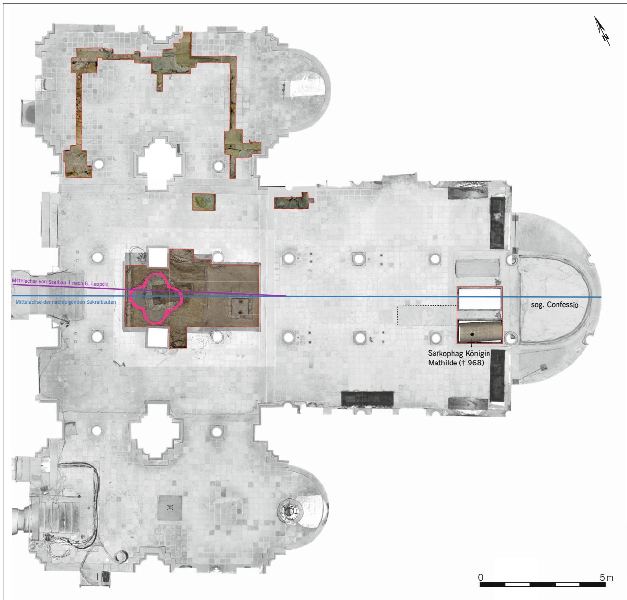
Abb. 27 Quedlinburg, St. Servatii. A 17364: Die Ausrichtung der Vierpassanlage im Verhältnis zur Mittelachse von Bau 1 nach Leopold und zur Mittelachse nachfolgender Kirchbauten (vgl. Abb. 28).
