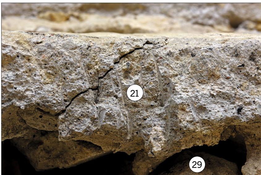
Abb. 17 Quedlinburg. Krypta St. Servatii. A 17364: Beim Einbau des gemauerten Schach- tes, Befund 22, wurden die Estrichdeckung der Phase 2 des Vierpasses, Befund 21, und das Füll- material, Befund 29, durchschlagen. Als Werk- zeug diente wohl ein Glattbeil. Dafür spricht die große Breite der ungeordneten scharfen Hiebe.
