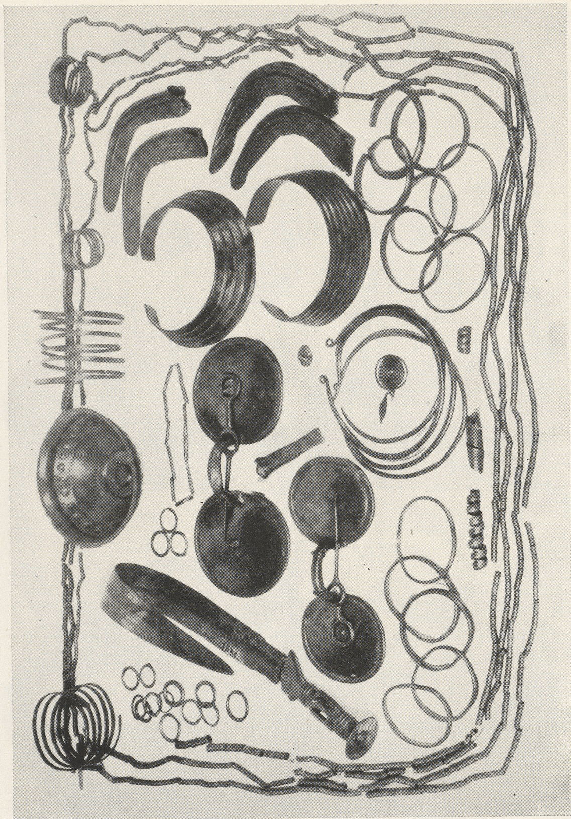
Quedlinburg-Lehof, Gesamtfund
