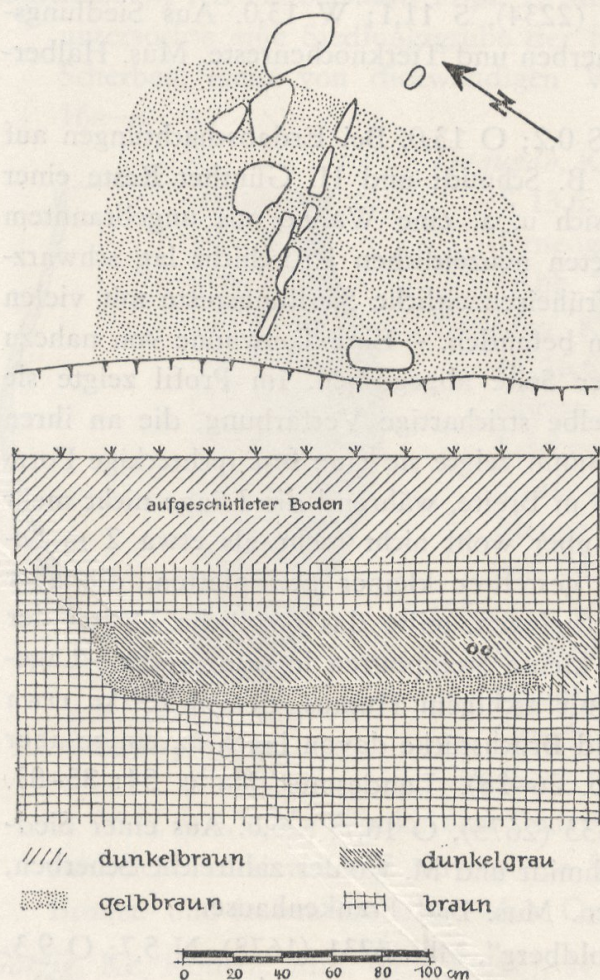
Abb. 26. Halle, Turbine-Sportplatz. Planum und Profil der Tonwanne.
